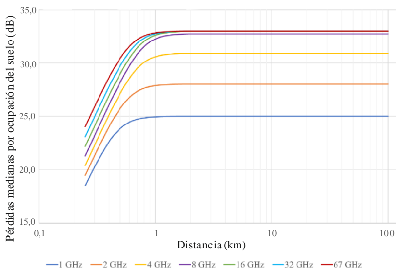
FIGURA 1 Pérdidas medianas por ocupación del suelo para trayectos terrenales
