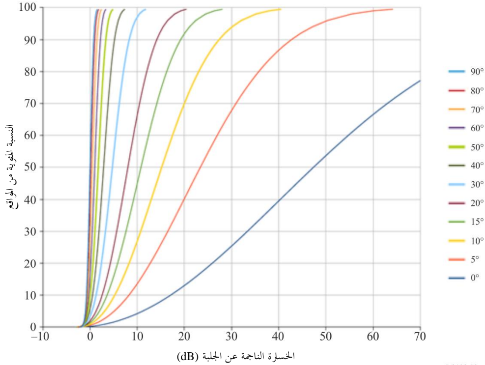
التوزيع التراكمي للخسارة الناجمة عن الجلبة التي لم تُتجاوز على تردد 30 GHz
