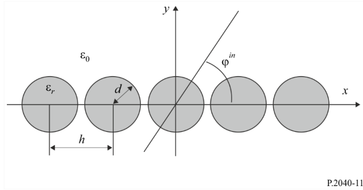
图11 一个周期性圆柱体阵列的几何图形
