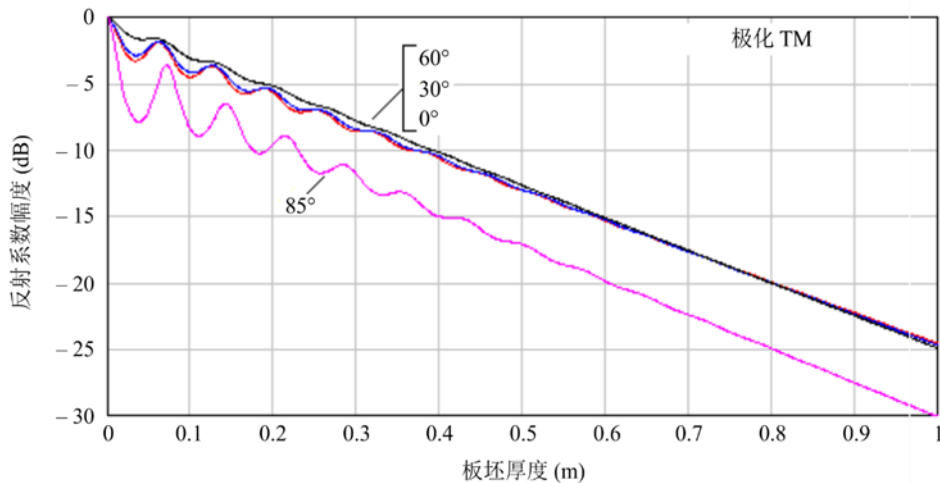
图7 在1 GHz的混凝土板坯透射系数，TM极化
