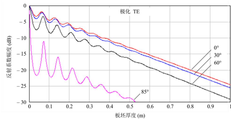
图6 在1 GHz的混凝土板坯透射系数，TE极化
