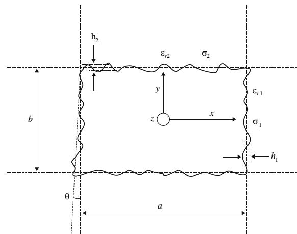
Поперечное сечение волновода и постоянные материалов
