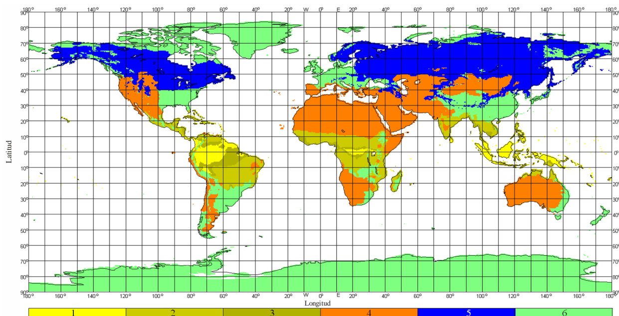
FIGURA E.1 Zonas climáticas
