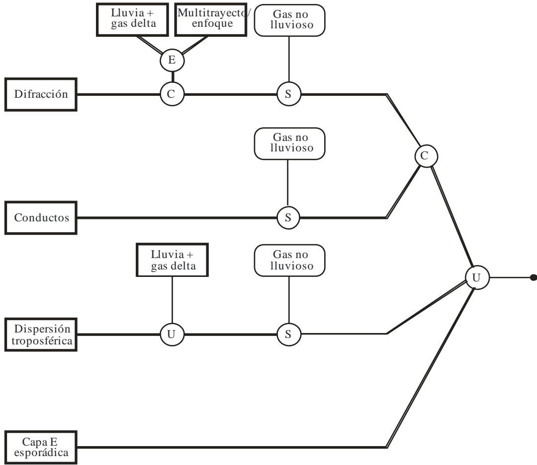
FIGURA J.2.1 Diagrama de combinación de los submodelos
