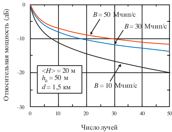
РИСУНОК 2 Профиль групповой задержки лучей PDP_{NLoS,env}(i, d) для условий NLoS
