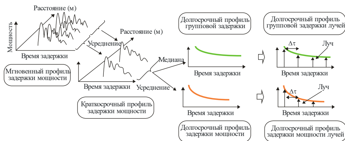
РИСУНОК 1 Профили задержки
