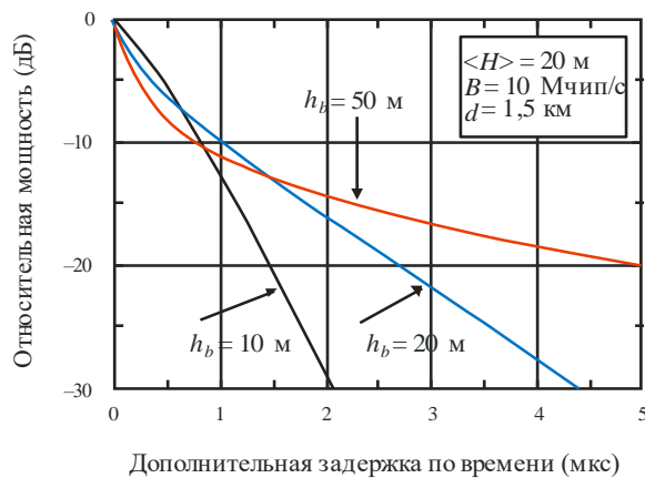
РИСУНОК 3 Профиль групповой задержки PDP_{NLoS,env}(\tau, d) для условий NLoS
