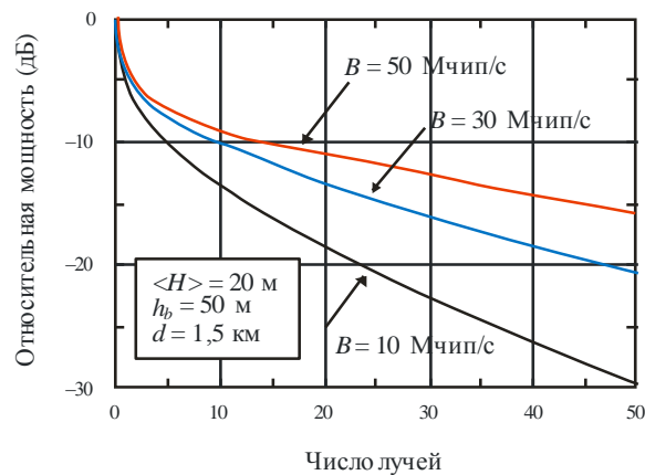
Профиль задержки мощности луча PDP_{NLoS, pow}(i, d) для условий NLoS
