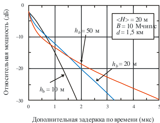
Профиль задержки мощности PDP_{NLoS, pow}(\tau, d) для условий NLoS
