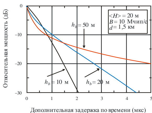
Профиль групповой задержки PDP_{NLoS,env}(\tau, d) для условий NLoS
