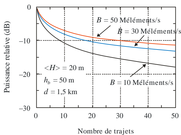
Profil d'enveloppe en fonction du retard de trajet PDP_{NLoS,env}(i, d) pour des environnements NLoS
