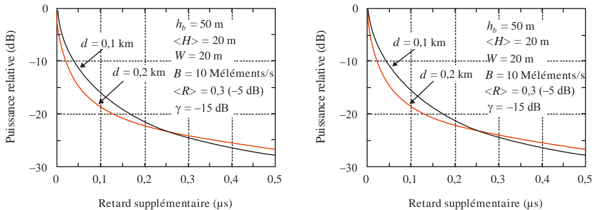
Profil d'enveloppe en fonction du retard PDP_{LoS,env}(\tau, d) pour des environnements LoS
