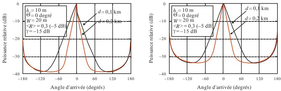
(a) Station de base faisant face au côté gauche ou droit de la rue (b) Station de base faisant face à l'extrémité de la rue
