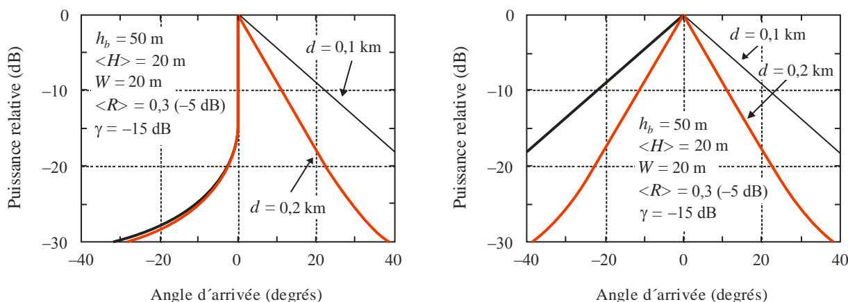
Profil de l'angle d'arrivée au niveau de la station de base AOD_{LoS,pow}(\Delta\theta, d) pour des environnements LoS
