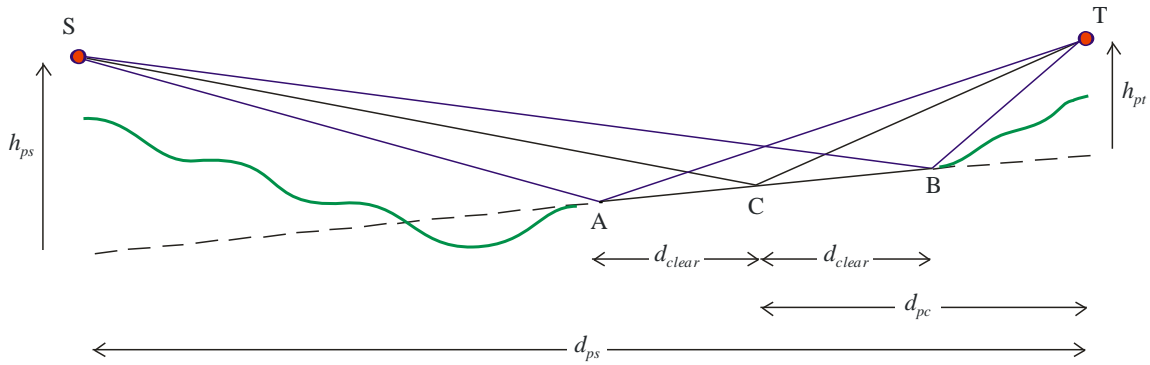
FIGURE 3 Géométrie requise pour les réflexions sur le sol
