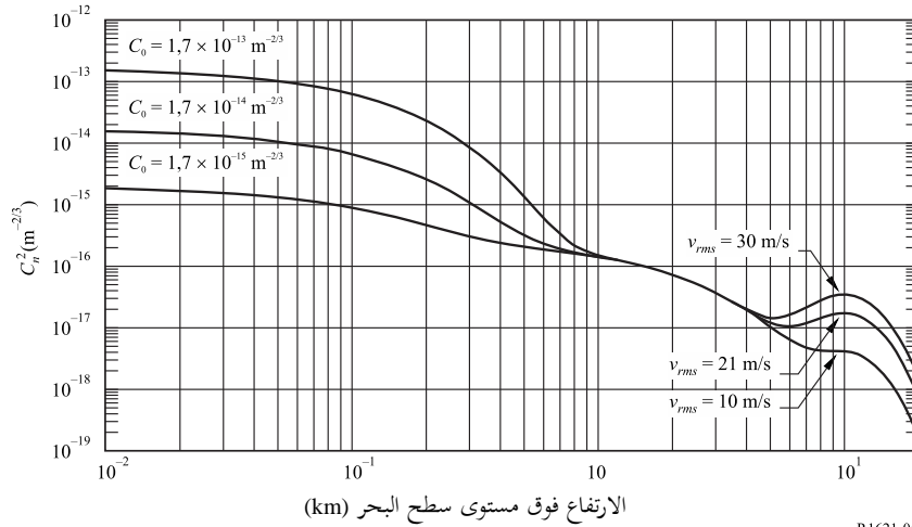
المعلمة C_n^2 كدالة ارتفاع لقيم متعددة لسرعة الرياح واضطراب السطح
