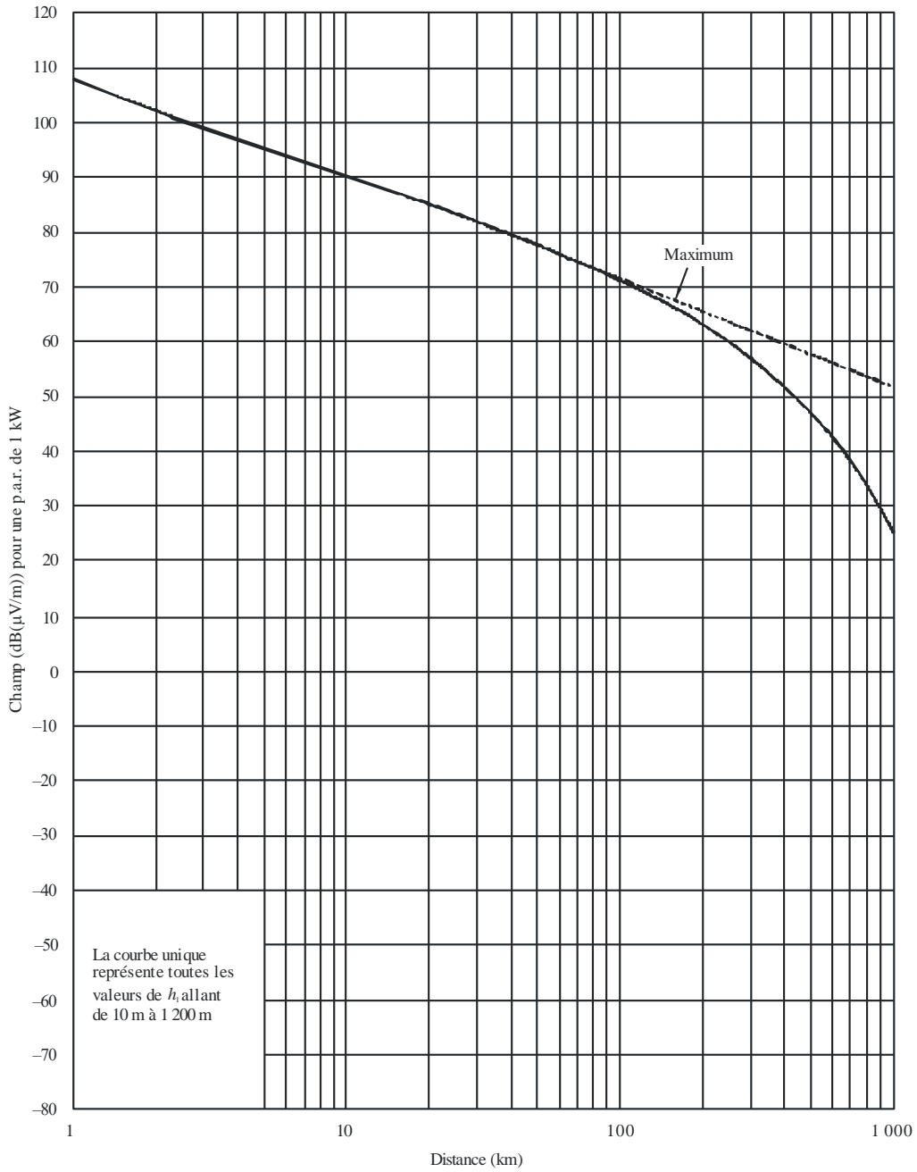
FIGURE 24 2 000 MHz, trajet mer chaude, 1% du temps
