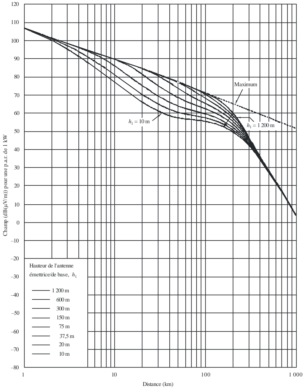
FIGURE 14 600 MHz, trajet mer froide, 1% du temps
