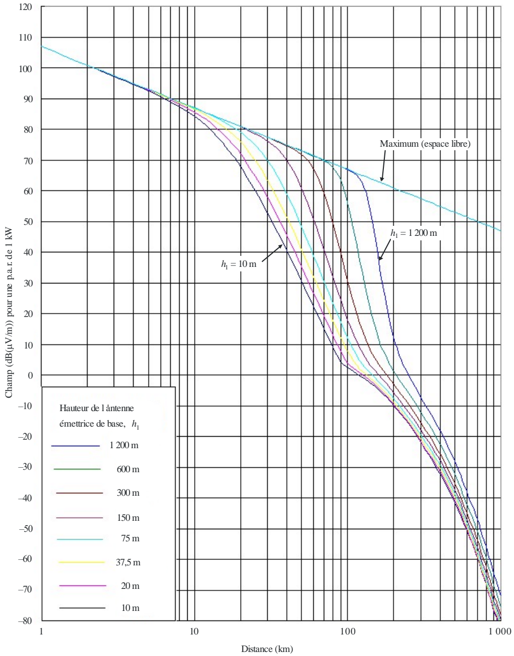
FIGURE 20 2 000 MHz, trajet maritime, 50% du temps
