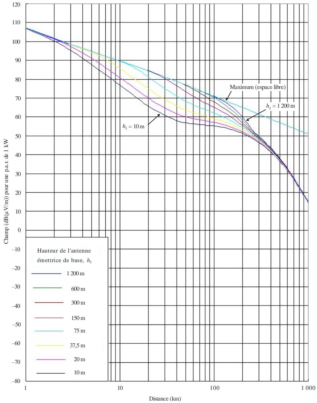
FIGURE 16 600 MHz, trajet mer chaude, 1% du temps
