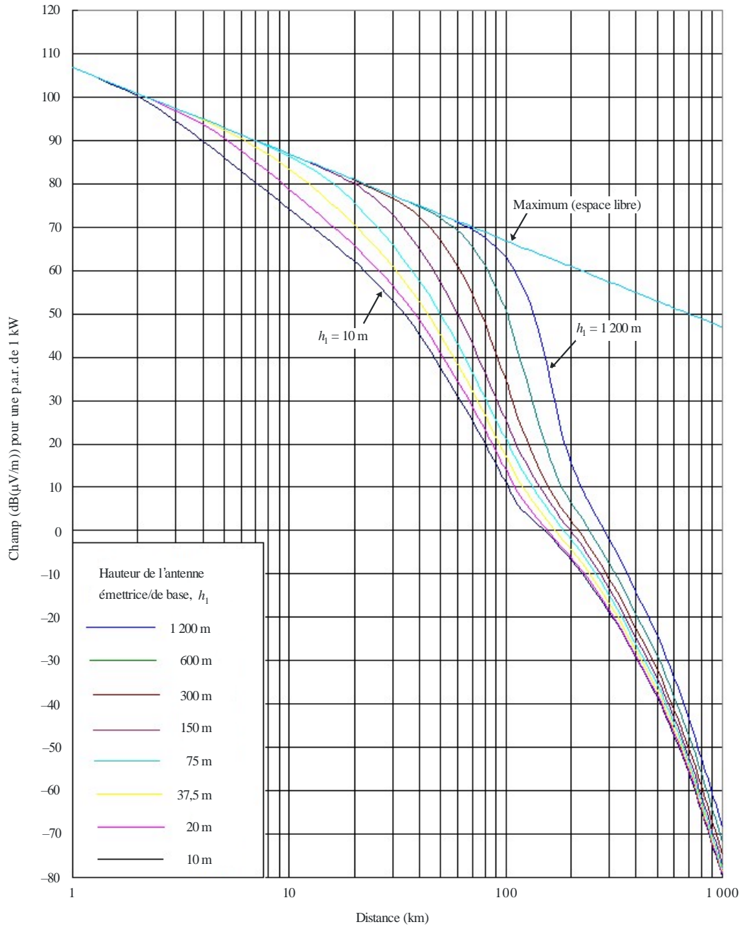
FIGURE 12 600 MHz, trajet maritime, 50% du temps
