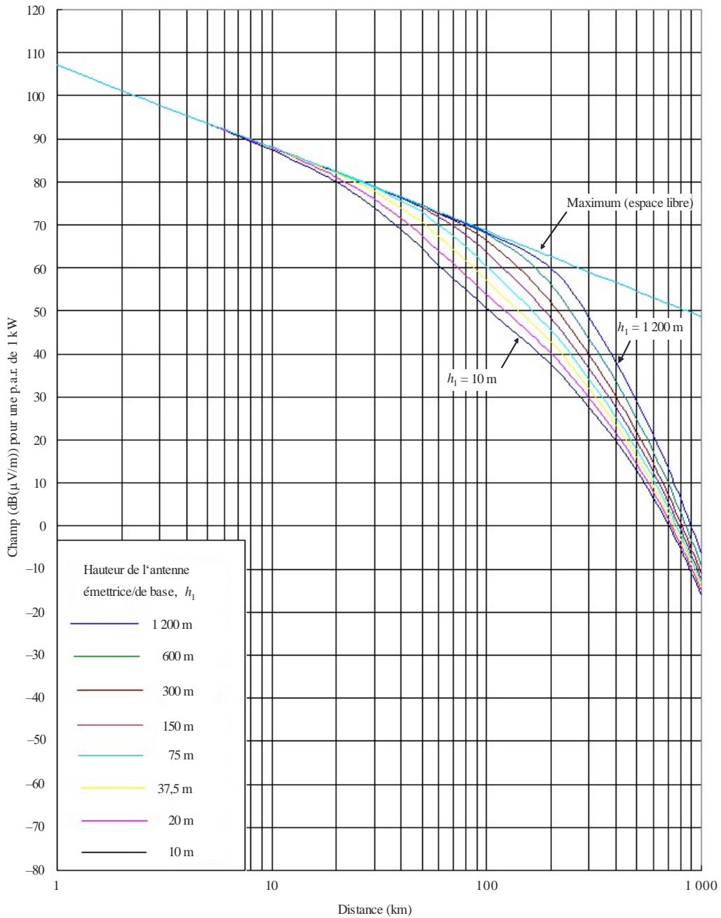
FIGURE 23 2 000 MHz, trajet mer chaude, 10% du temps
