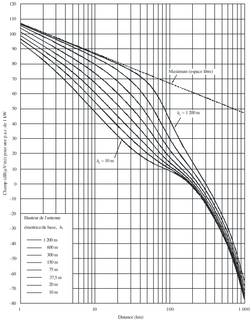
FIGURE 18 2 000 MHz, trajet terrestre, 10% du temps
