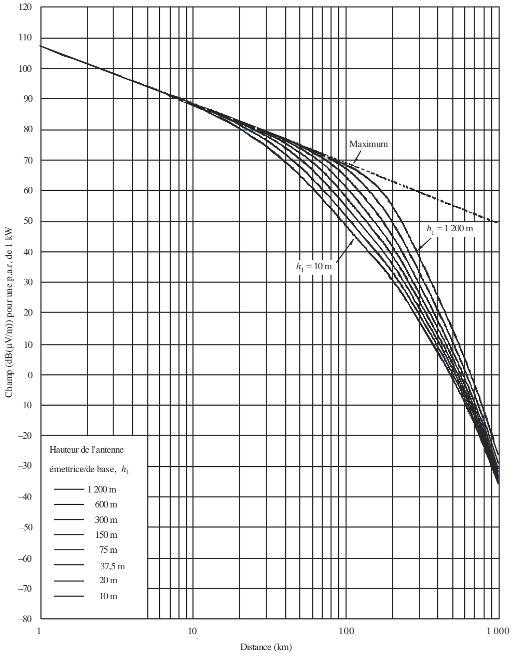
FIGURE 21 2 000 MHz, trajet mer froide, 10% du temps
