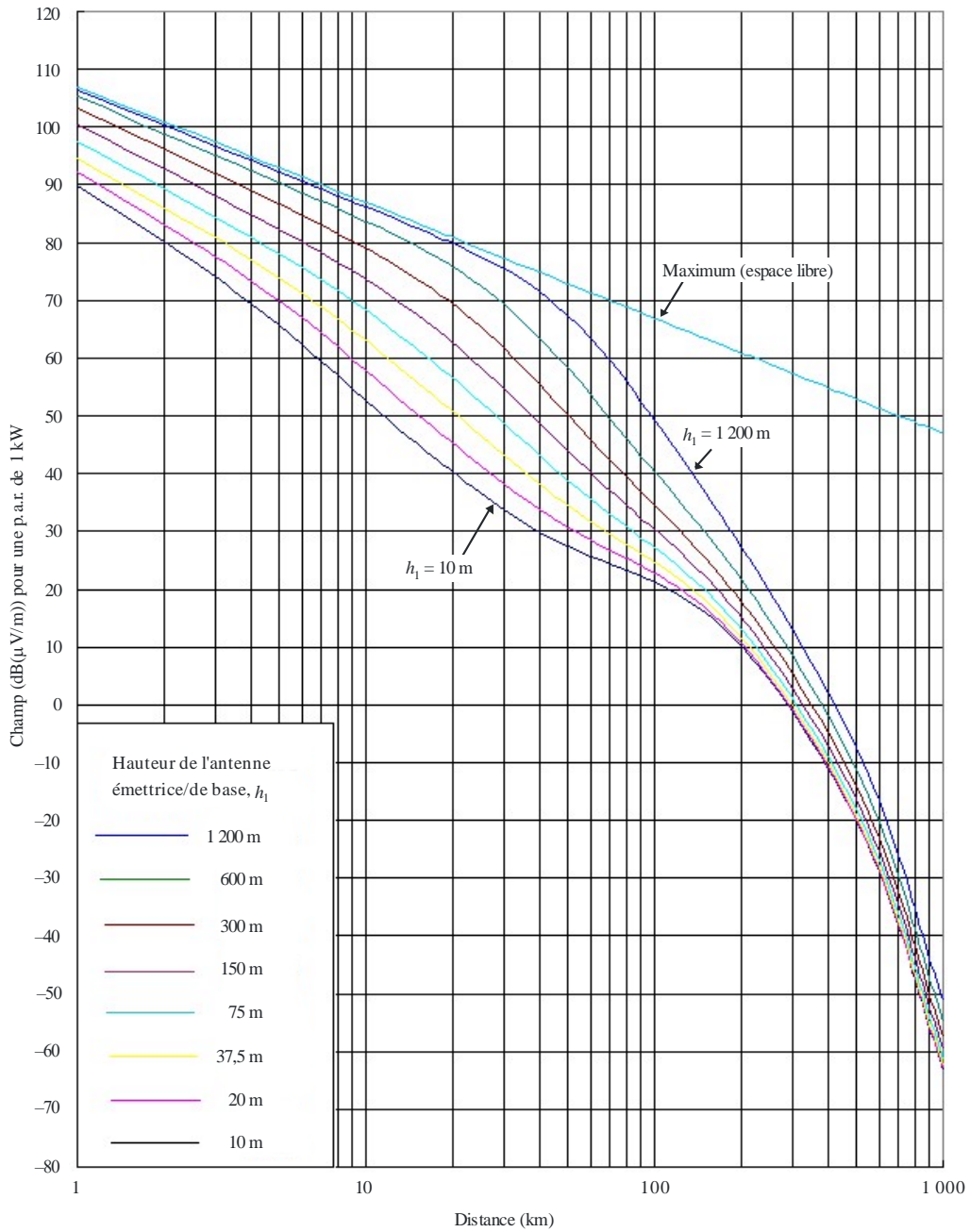
FIGURE 2 100 MHz, trajet terrestre, 10% du temps
