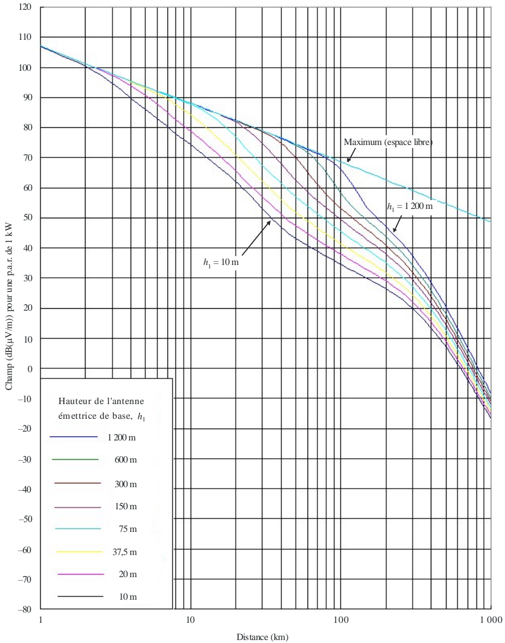
FIGURE 15 600 MHz, trajet mer chaude, 10% du temps
