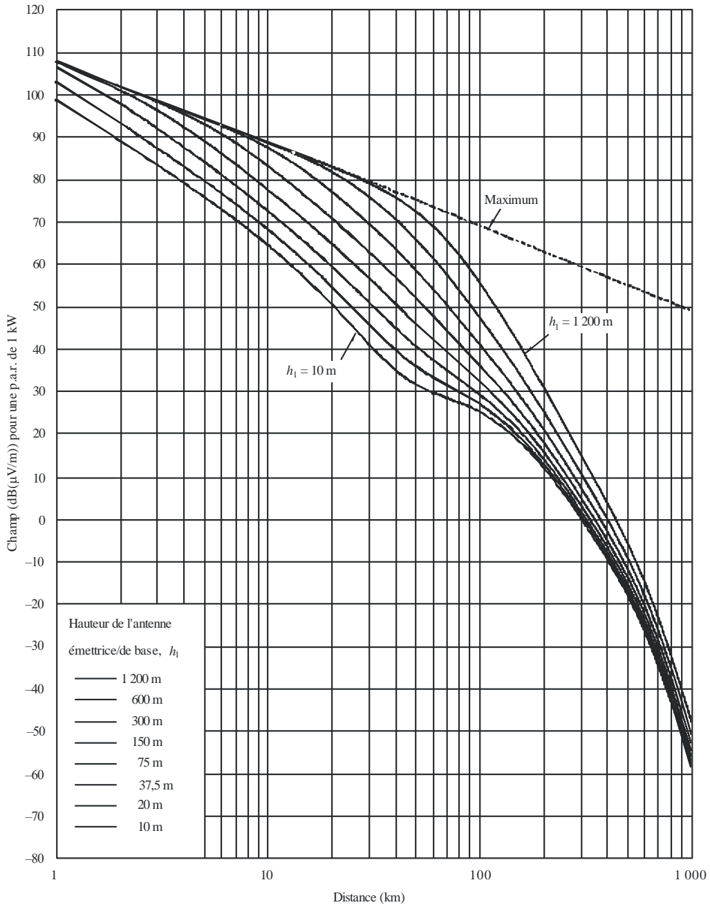
FIGURE 5 100 MHz, trajet mer froide, 10% du temps
