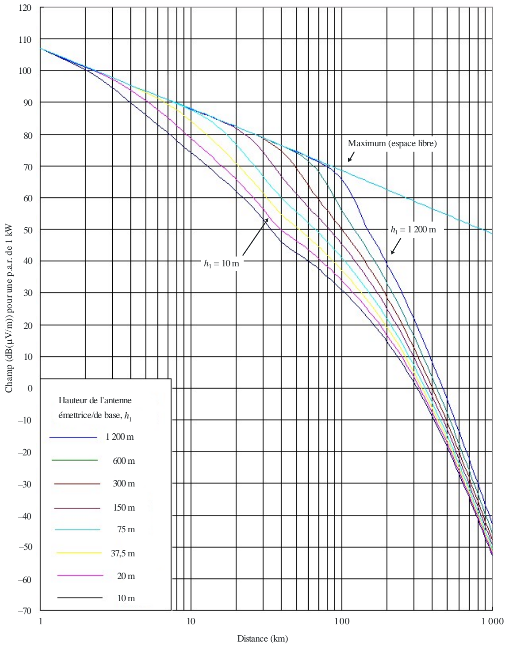
FIGURE 13 600 MHz, trajet mer froide, 10% du temps
