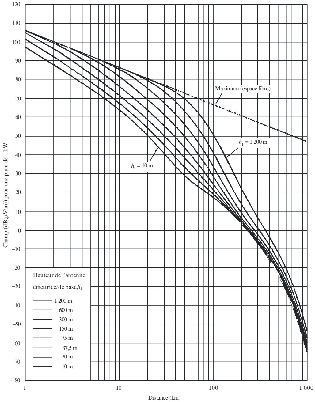
FIGURE 4 100 MHz, trajet maritime, 50% du temps
