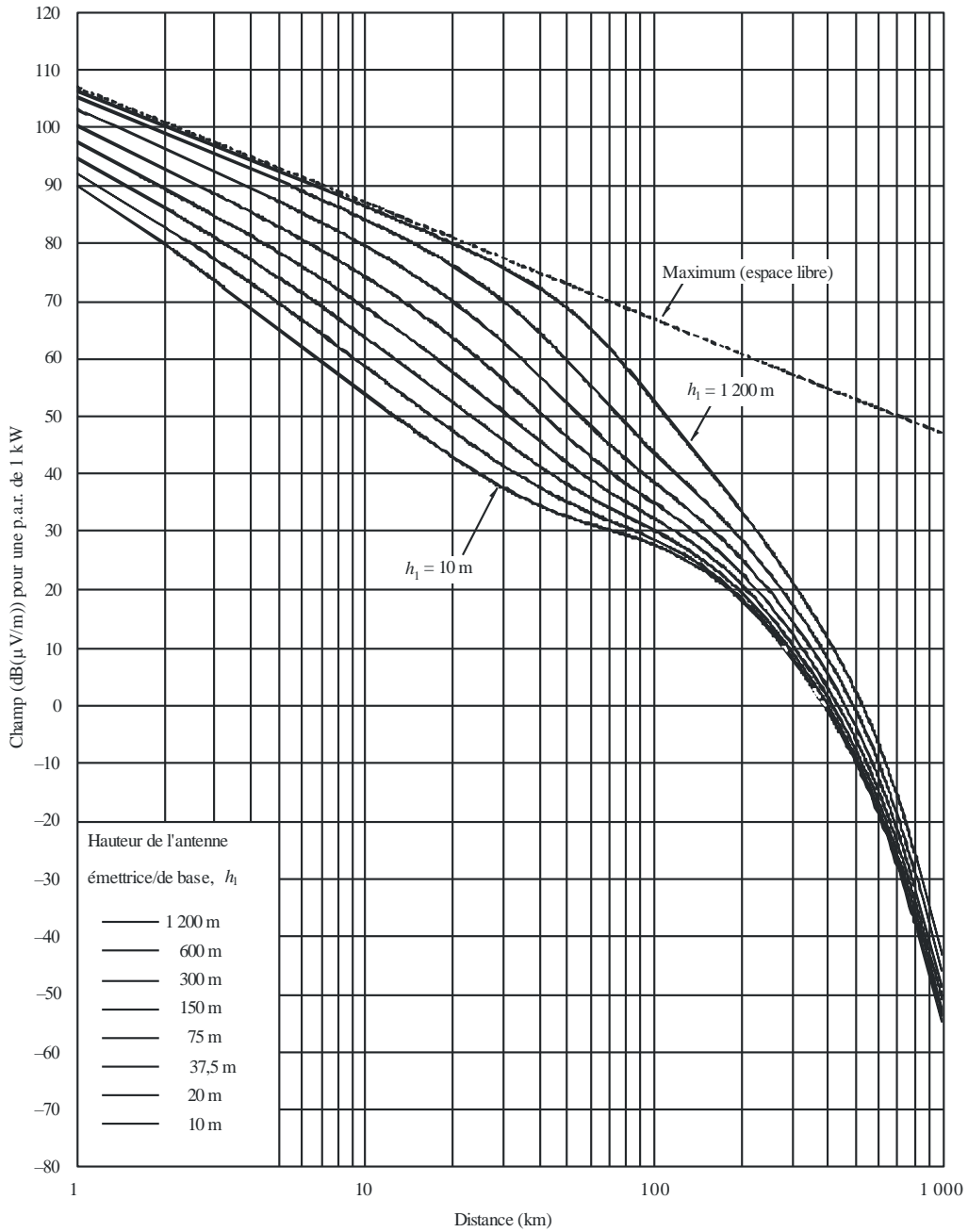
FIGURE 3 100 MHz, trajet terrestre, 1% du temps
