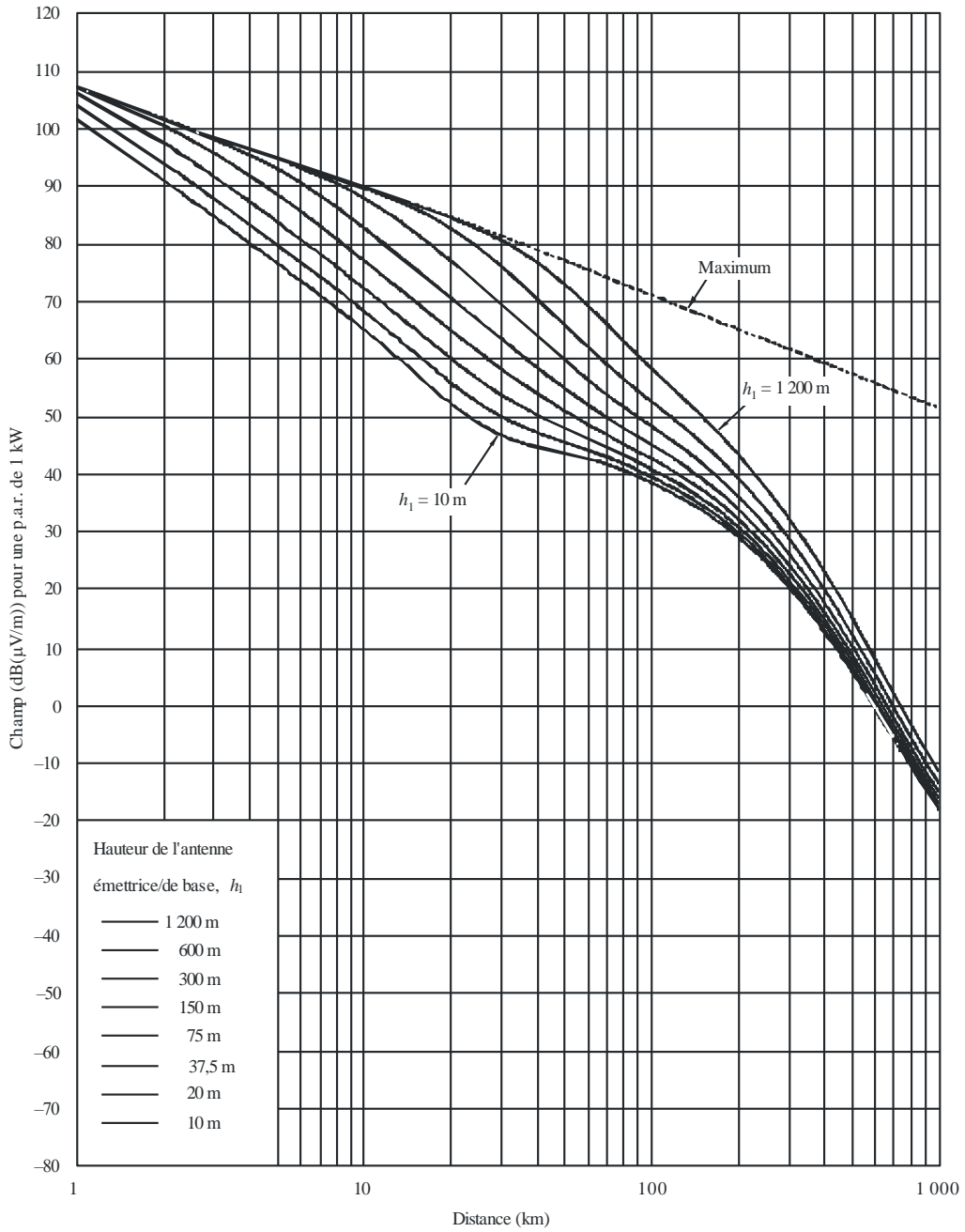
FIGURE 6 100 MHz, trajet mer froide, 1% du temps
