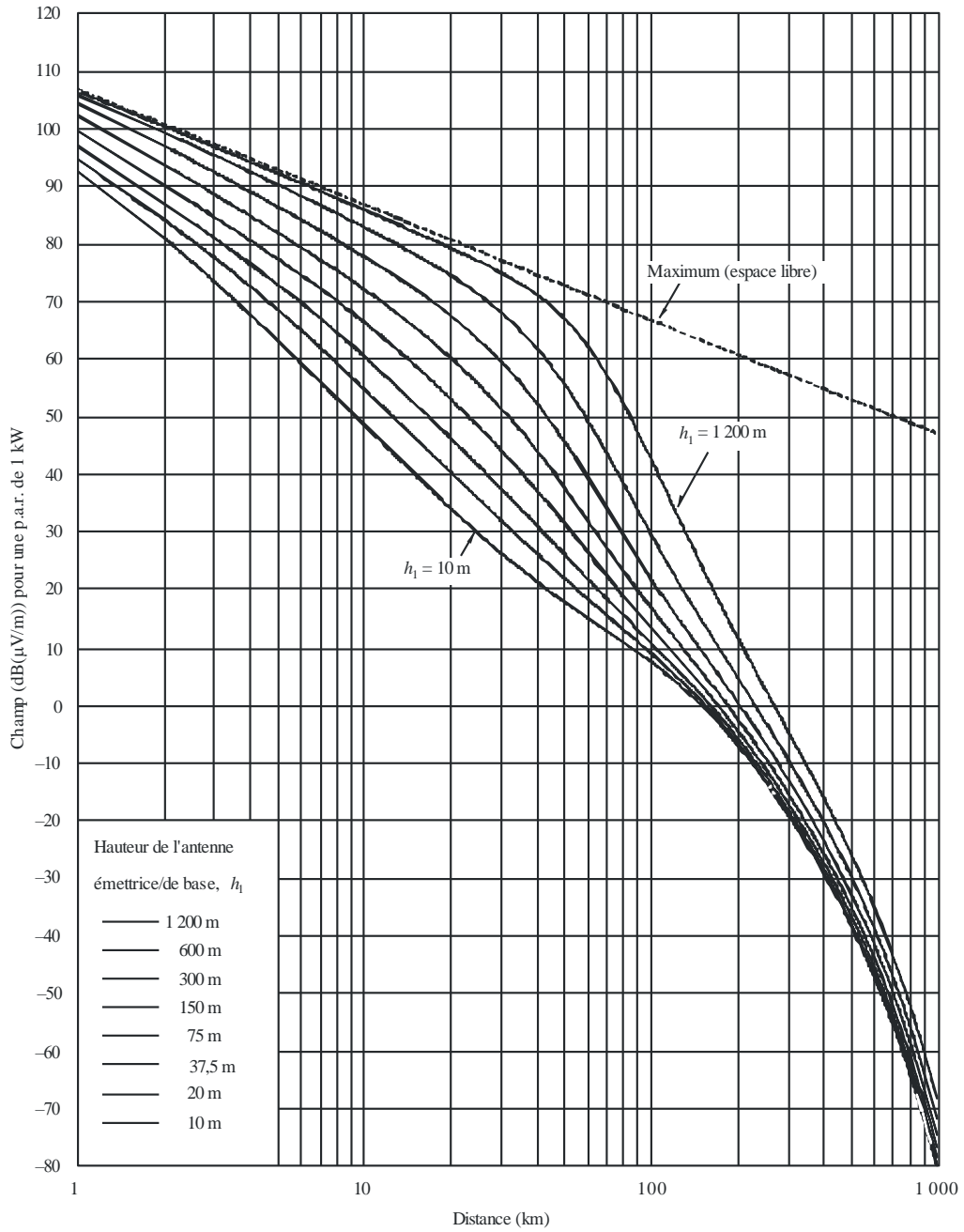
FIGURE 9 600 MHz, trajet terrestre, 50% du temps
