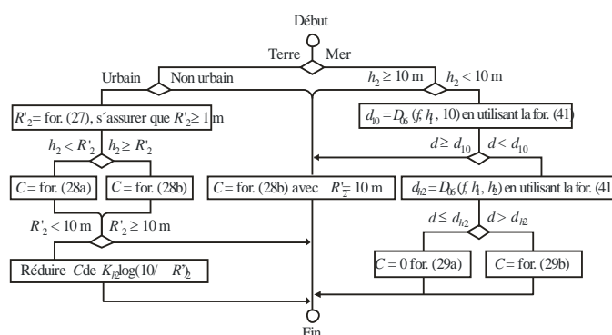
FIGURE 27 Diagramme pour la correction liée à la hauteur de l'antenne réceptrice/mobile
