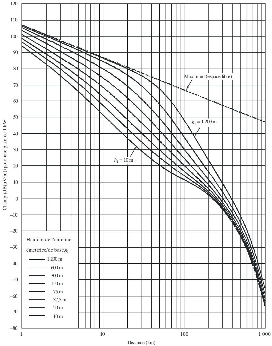
FIGURE 19 2 000 MHz, trajet terrestre, 1% du temps
