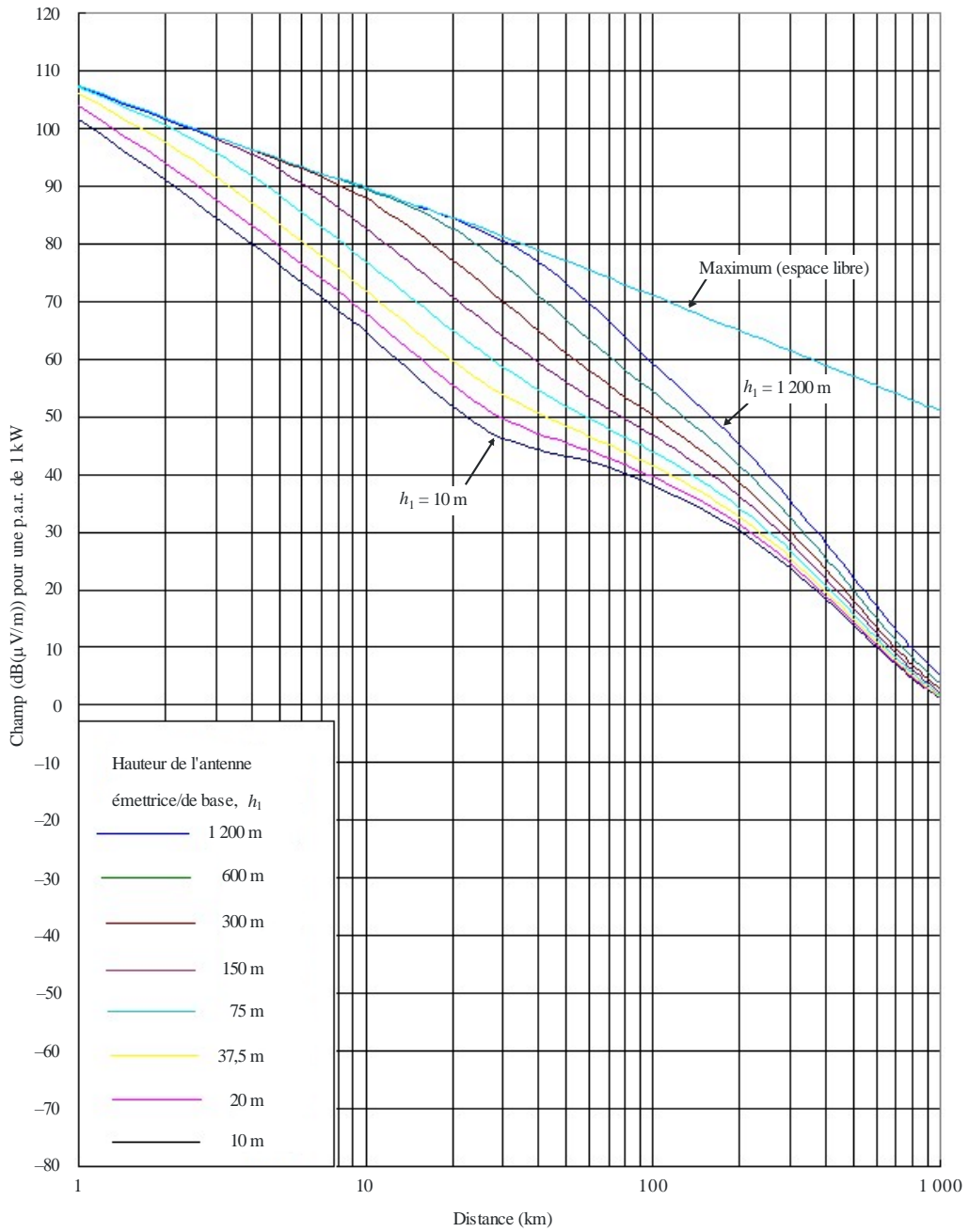
FIGURE 8 100 MHz, trajet mer chaude, 1% du temps
