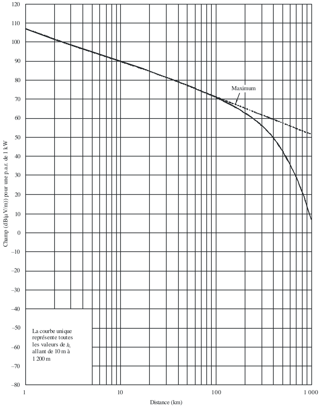
FIGURE 22 2 000 MHz, trajet mer froide, 1% du temps
