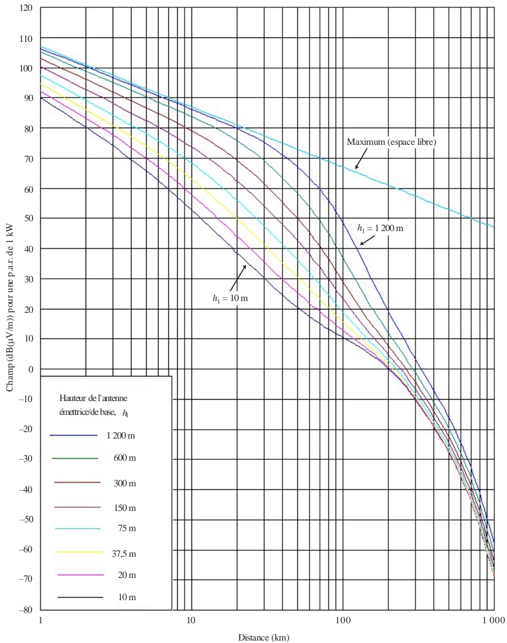
FIGURE 1 100 MHz, trajet terrestre, 50% du temps
