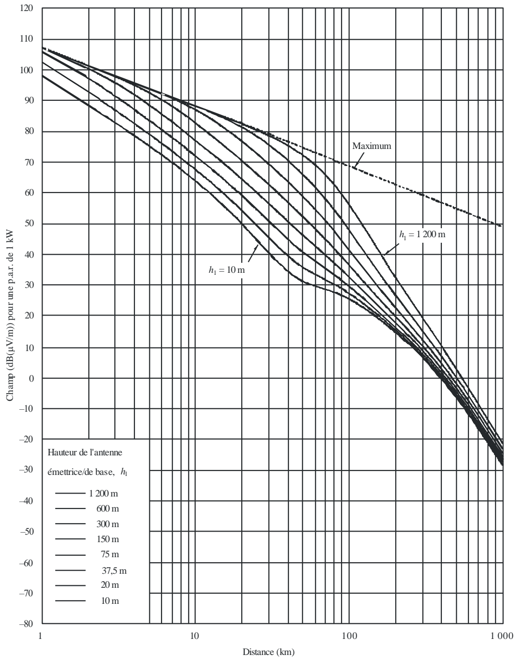
FIGURE 7 100 MHz, trajet mer chaude, 10% du temps
