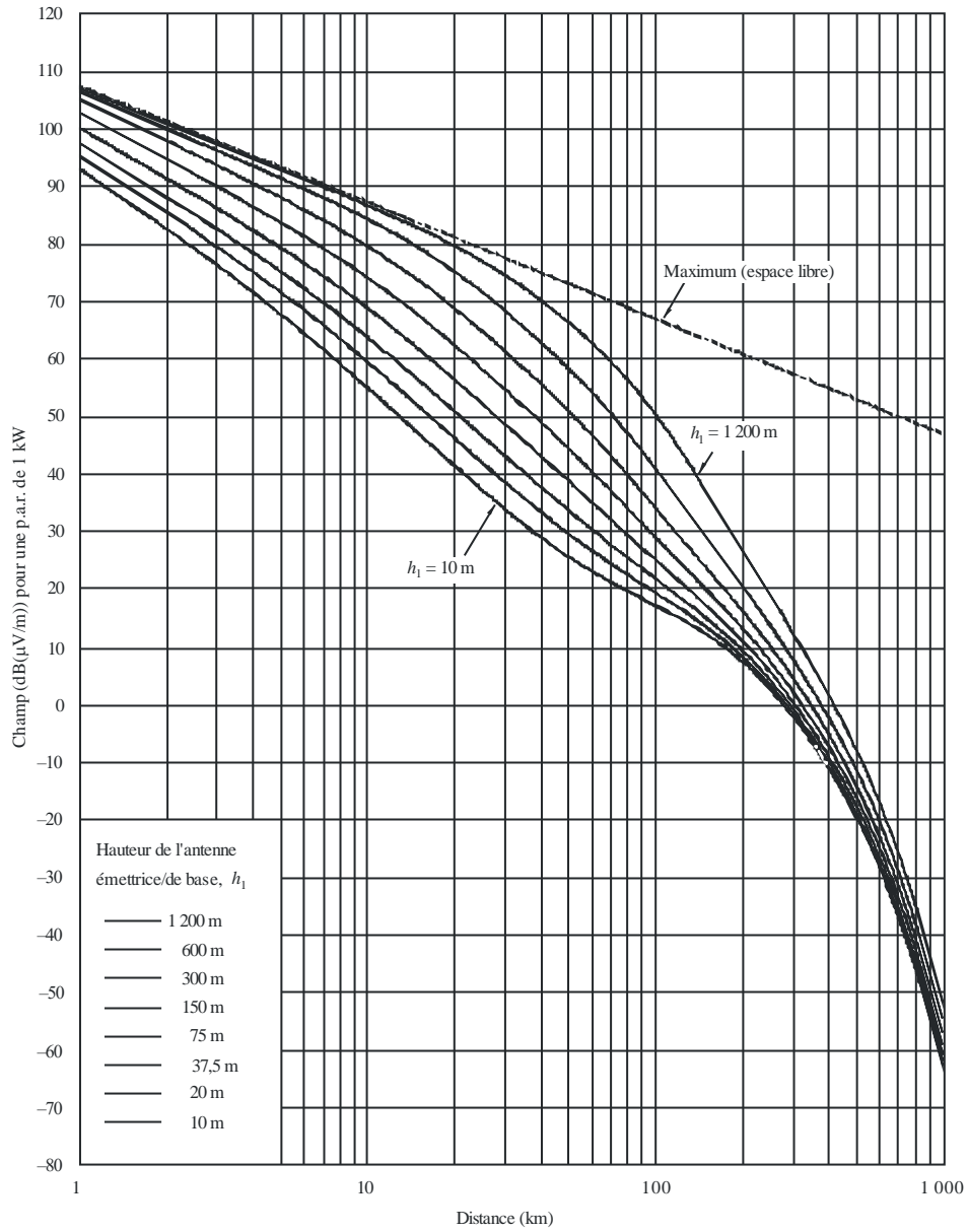
FIGURE 11 600 MHz, trajet terrestre, 1% du temps
