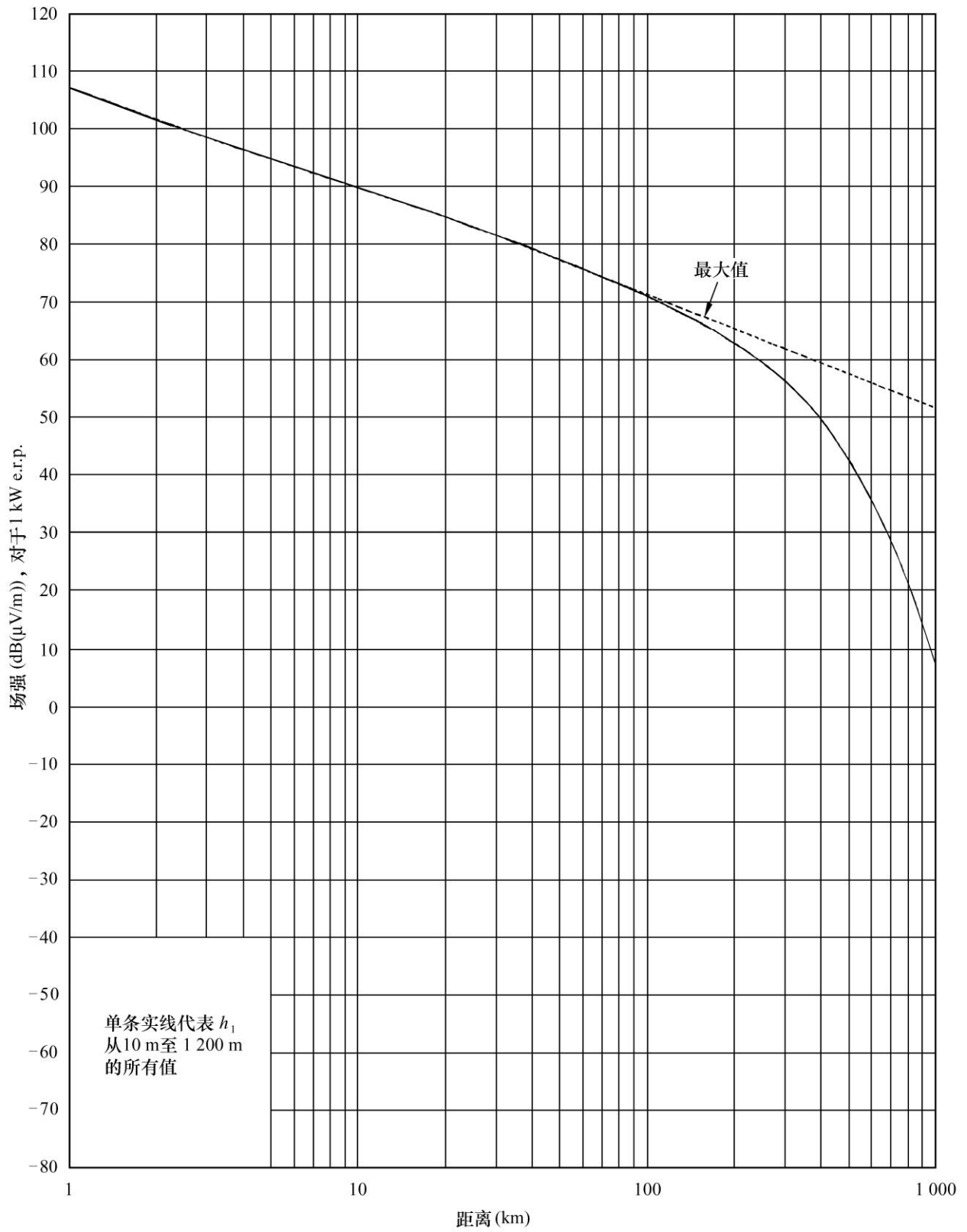
2 000 MHz, 冷海路径, 1%时间
