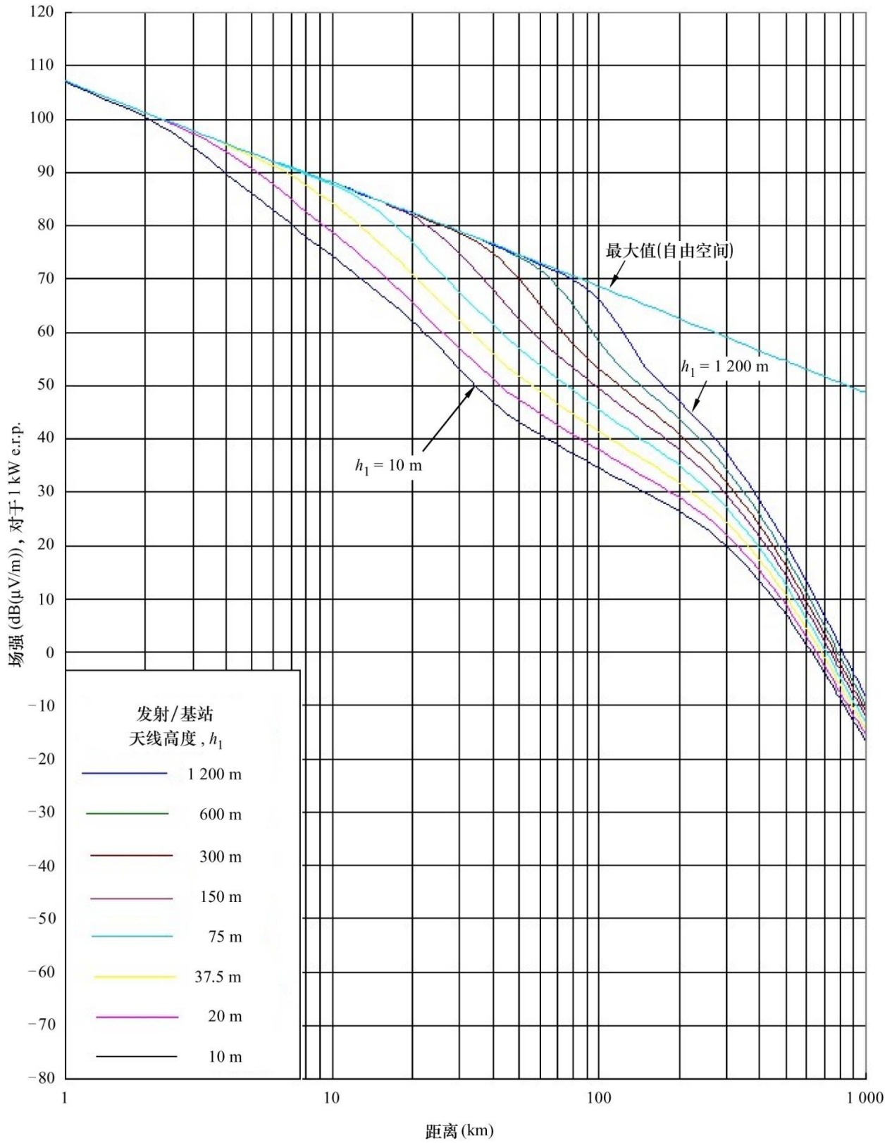
600 MHz, 暖海路径, 10%时间
