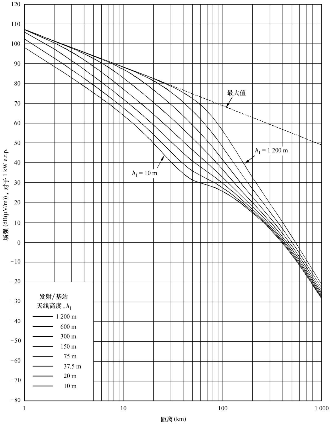
100 MHz, 暖海路径, 10%时间
