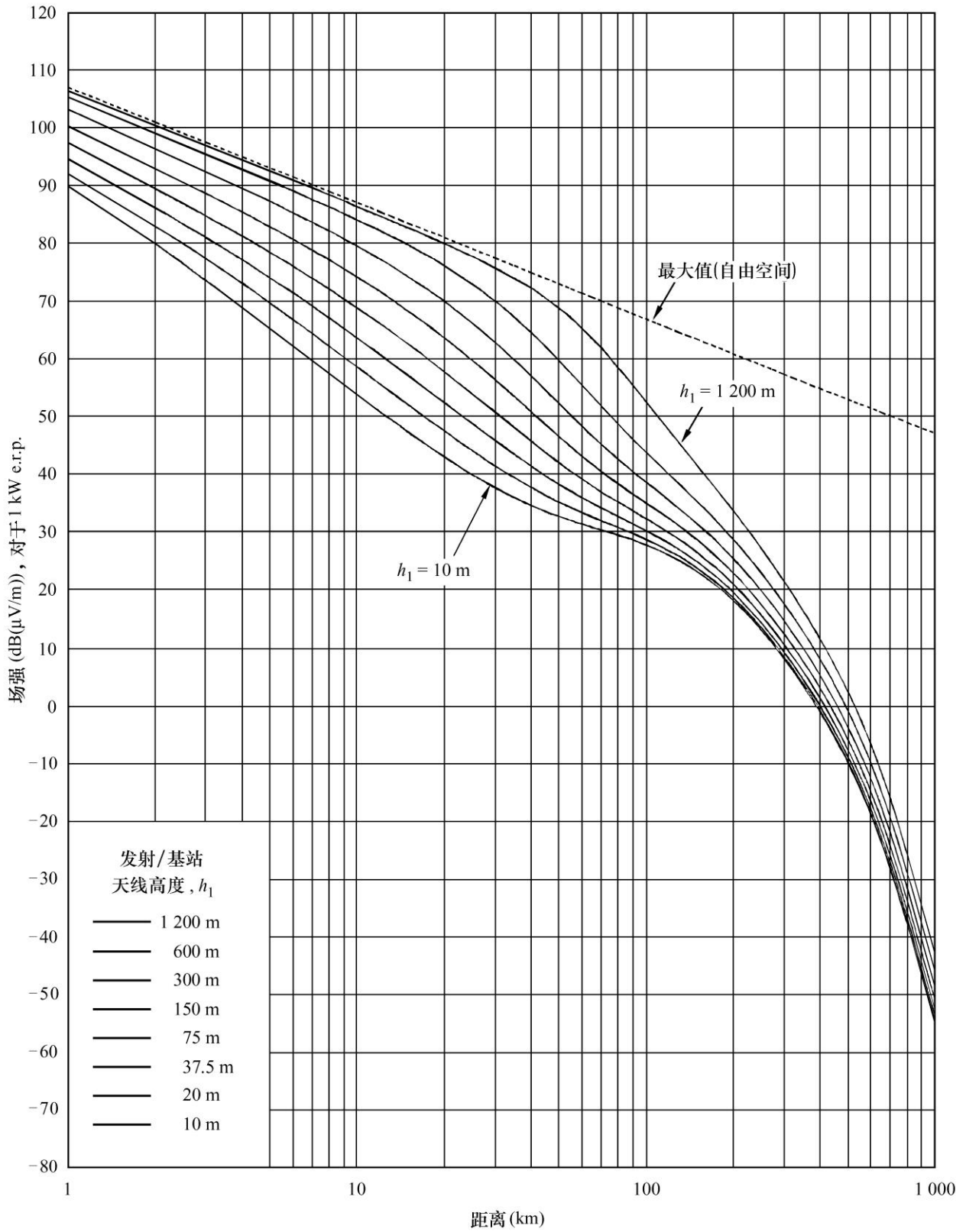
图3 100 MHz, 陆地路径, 1%时间
