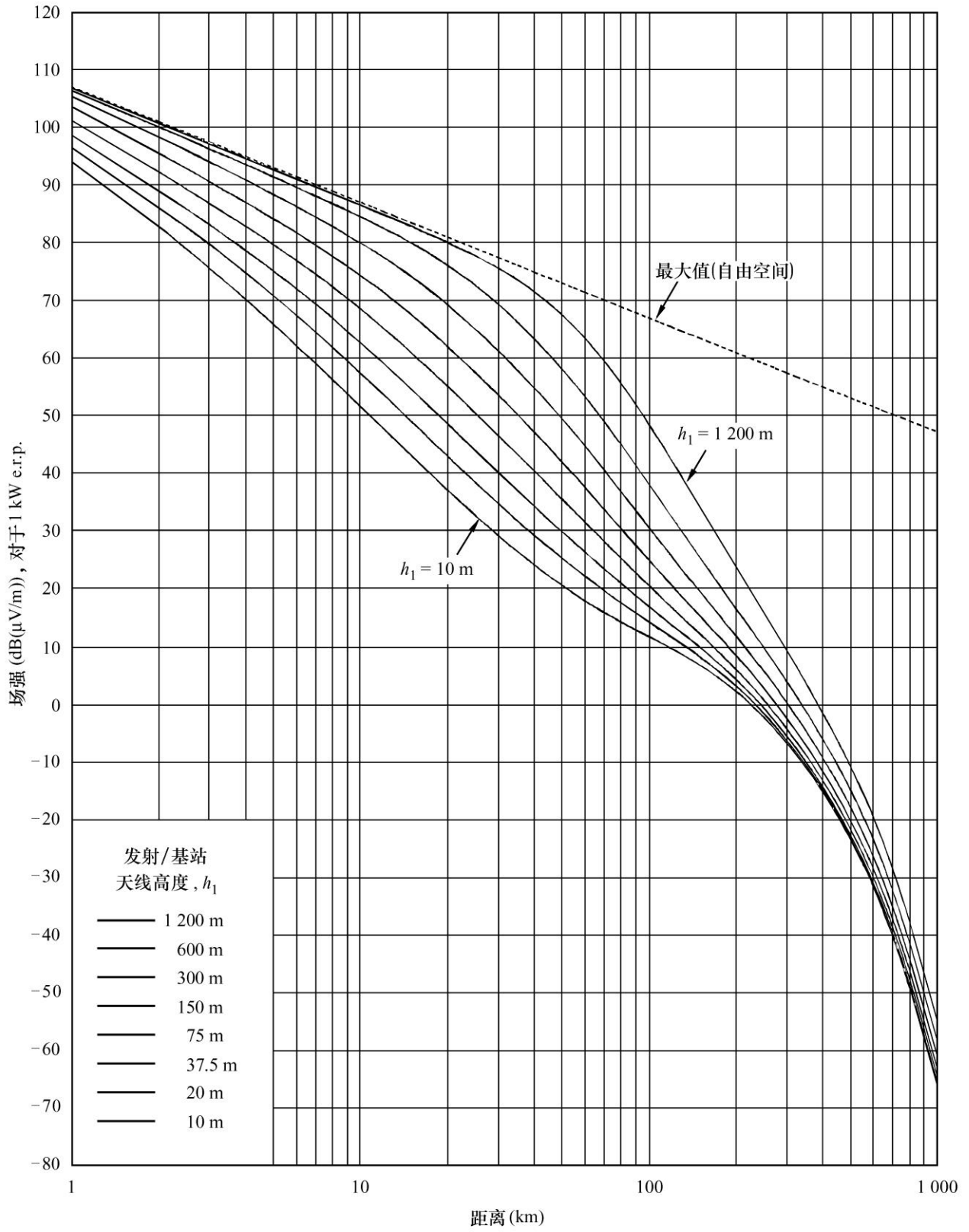
2 000 MHz, 陆地路径, 1%时间
