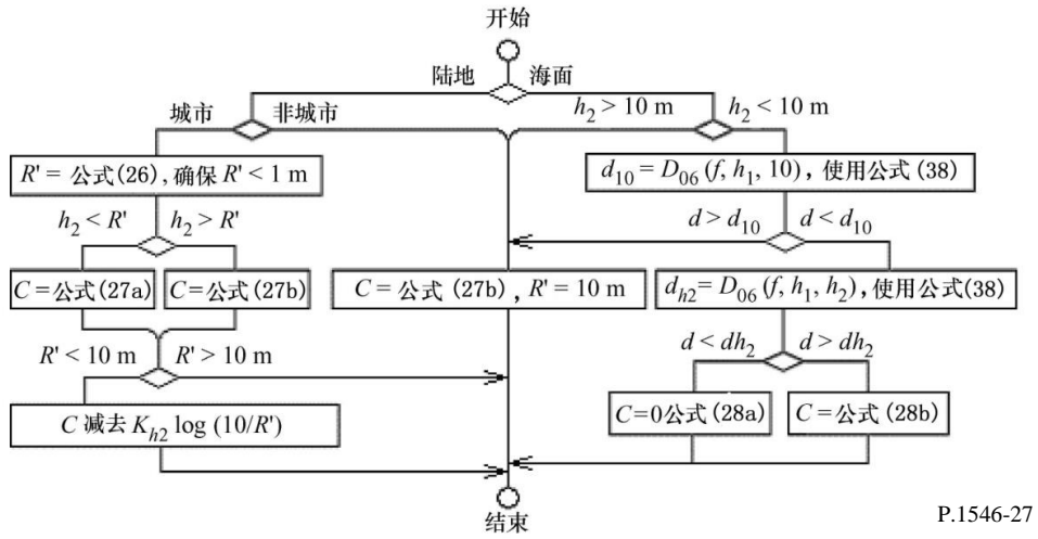
图27 接收/移动台天线高度校正项的计算流程图
