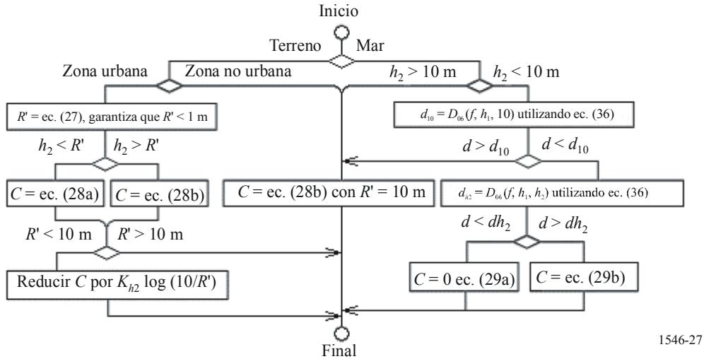
FIGURA 27 Organigrama para la corrección de altura de antena receptora/móvil
