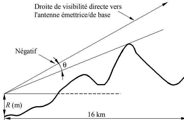
FIGURE 26b Angle de dégagement du terrain: cas où le trajet est en visibilité directe
