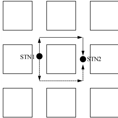
图8 2-turn NLoS路径的传输链路（实线和虚线）
