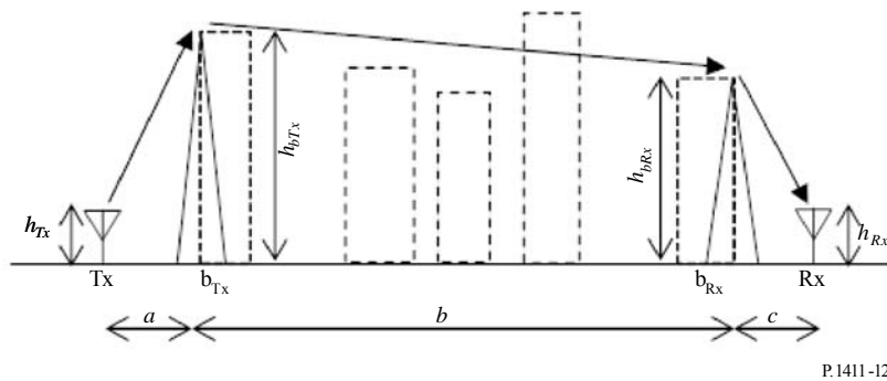
图12 建筑物几何图形和参数侧图
