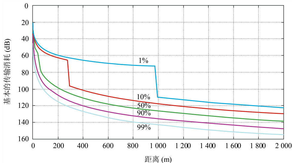
图6 不超过1%、10%、50%、90%和99%位置的基本传输损耗曲线 (频率=400 MHz, 郊区)
