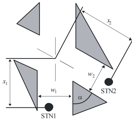
图3 NLoS2情况的参数定义
