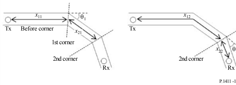
图11 道路几何图形和参数（以两个拐角为例）
