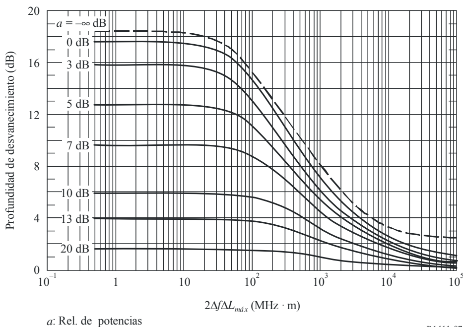
Relación entre la profundidad de desvanecimiento y 2\Delta f\Delta L_{m\acute{a}x}
