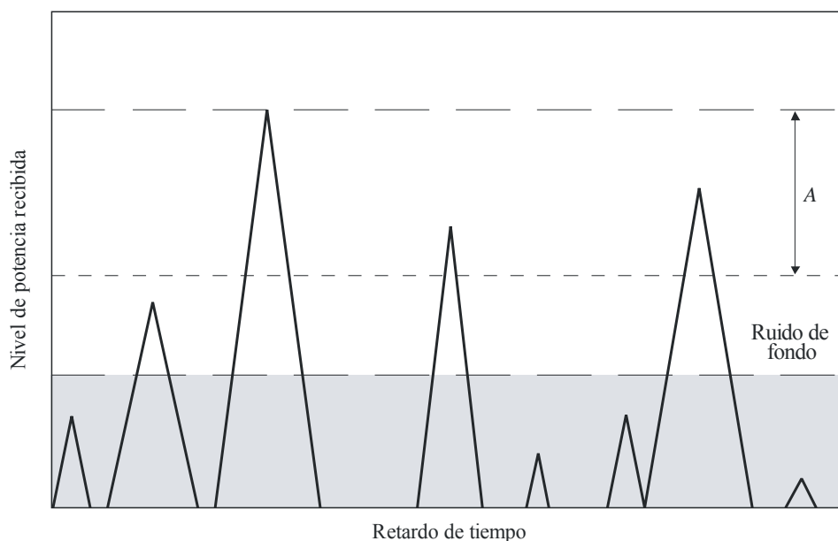
FIGURA 6 Definición para la determinación del número de crestas
