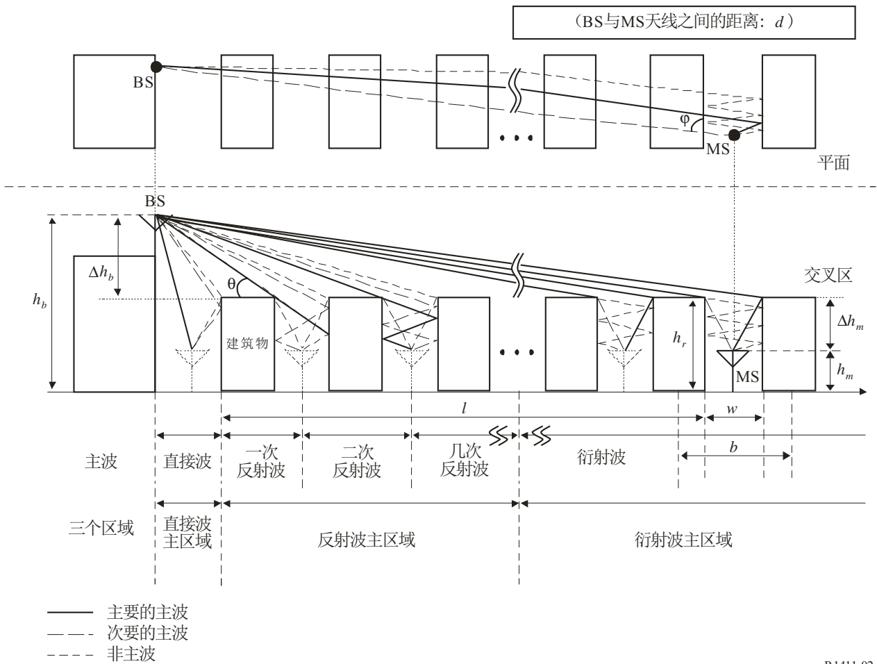
NLoS1情况下的参数定义
