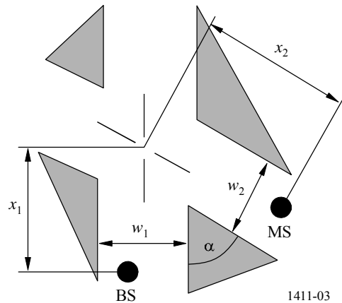
图3 对 NLoS2 情况的参数的规定
