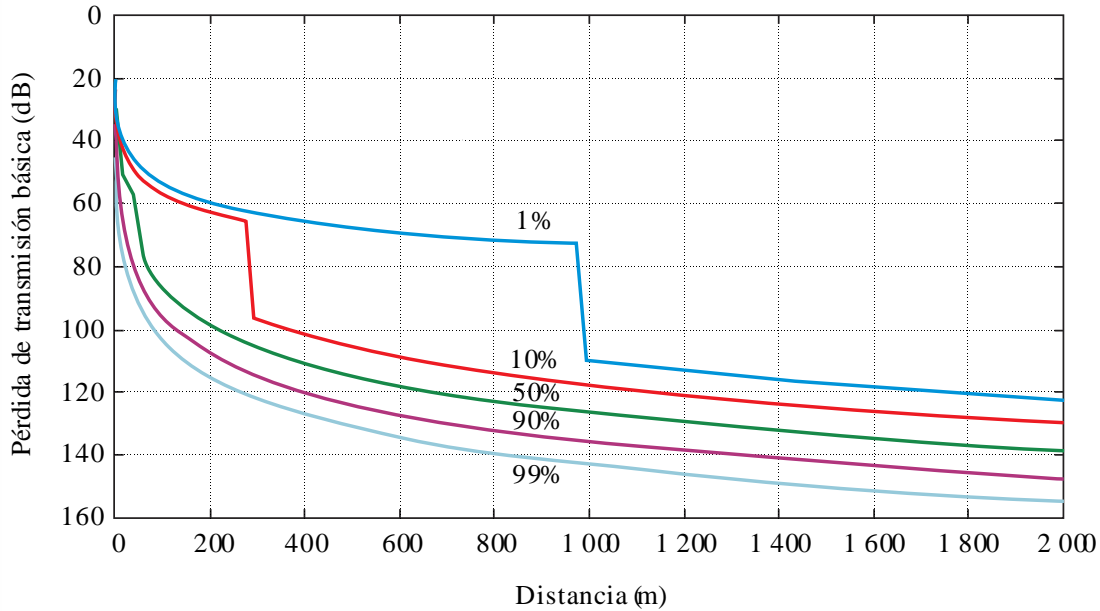
FIGURA 6 Curvas de pérdida de transmisión básica no excedidas en el 1, 10, 50, 90 y 99% de los emplazamientos (frecuencia = 400 MHz, entorno suburbano)
