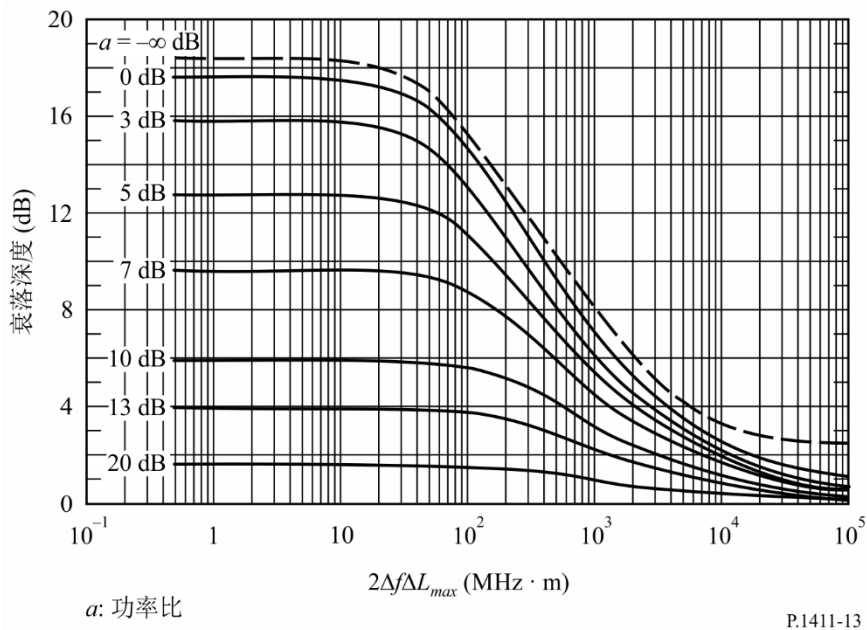
衰落深度和 2\Delta f\Delta L_{max} 之间的关系
