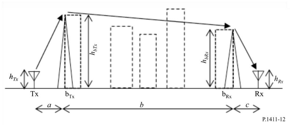
建筑物几何图形和参数侧图
