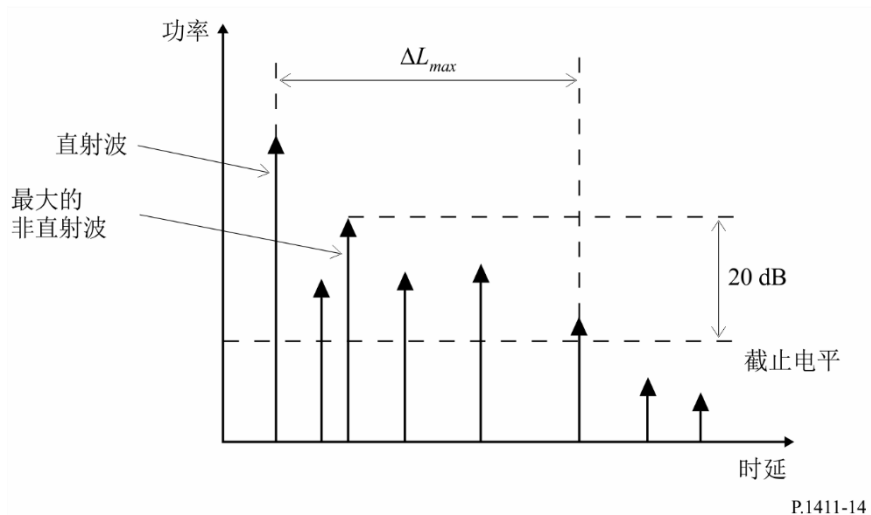
计算 \Delta L_{max} 的模型
