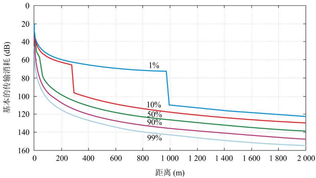
图6 不超过1%、10%、50%、90%和99%位置的基本传输损耗曲线 (频率=400 MHz, 郊区)
