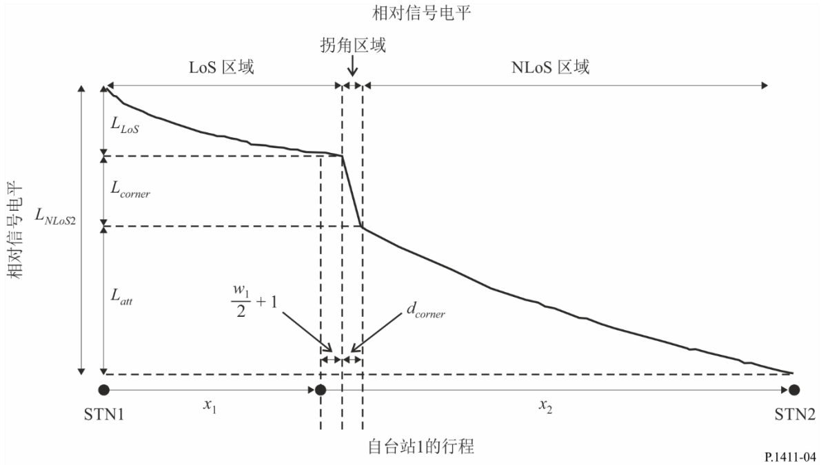
图4 2-38 GHz频率范围内低台站高度情况下 沿街道峡谷传播的典型趋势
