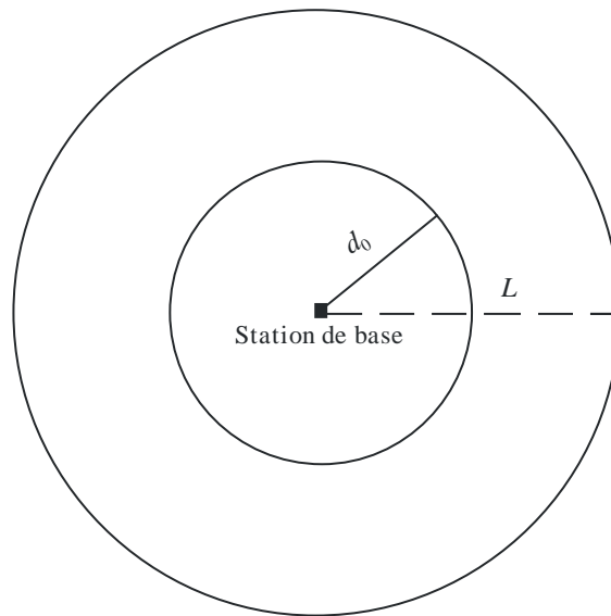
FIGURE 13 Schéma de la cellule à station centrale représentant le rayon de la zone de couverture équivalente durant les précipitations
