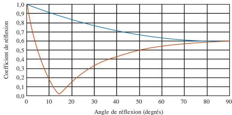
FIGURE 3 Coefficient de réflexion de Fresnel R_F parallèle (bleu) et perpendiculaire (rouge) en fonction de l'angle (3,5 GHz, surface sèche moyenne)
