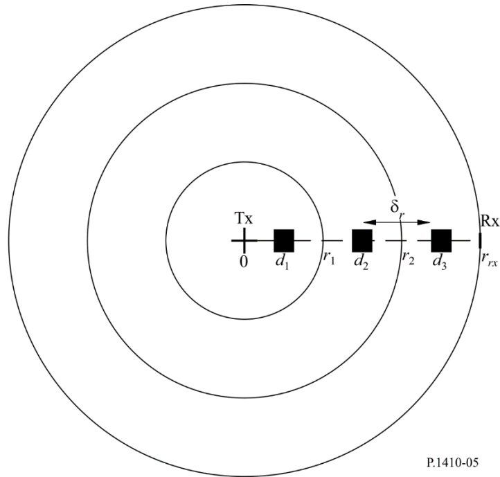
图5 有关Rx在距Tx r_{rx} 处的建筑物位置
