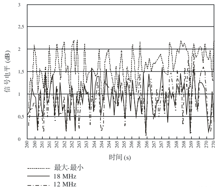
信道的信号电平在不同风速条件下的比较
