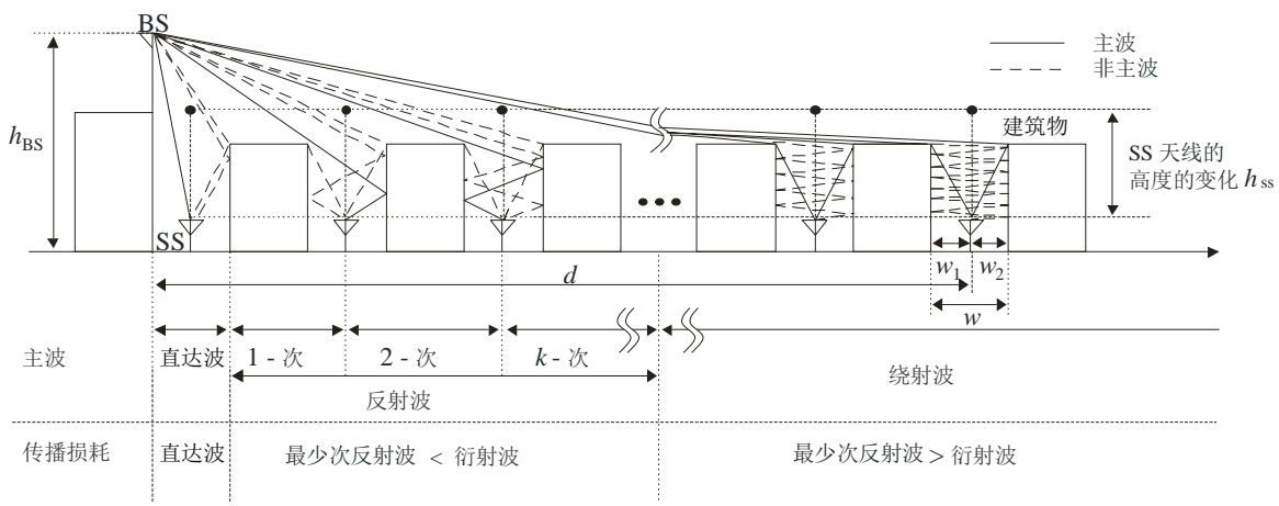
在几何传播模型基础上的屋顶上的传播机制
