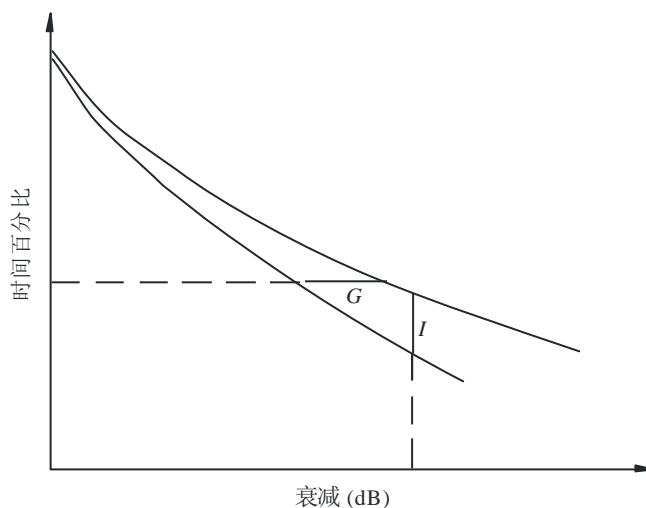
图15 路径-角度分集衰减统计的例子
