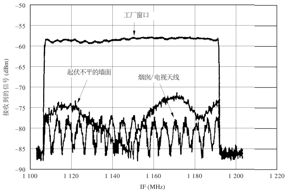
图 17 在三个不同位置测得的频率响应
