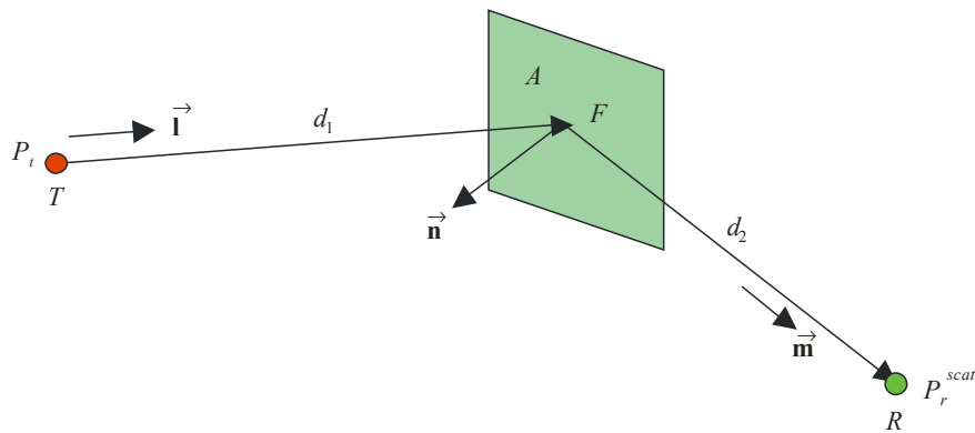
РИСУНОК 2 Геометрия отражения
