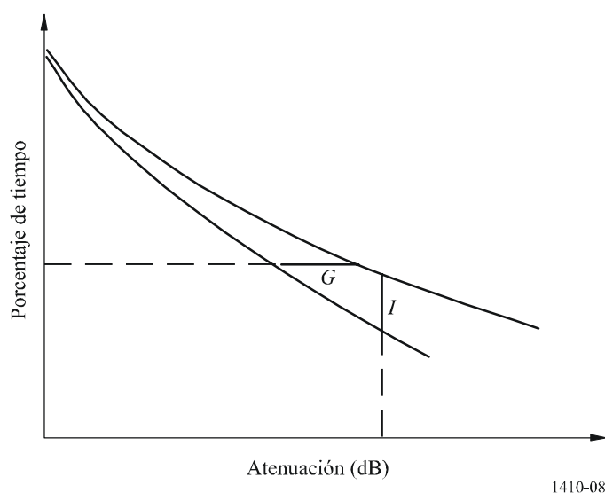
FIGURA 8 Ejemplo de estadísticas de atenuación con diversidad de ángulos de trayecto
