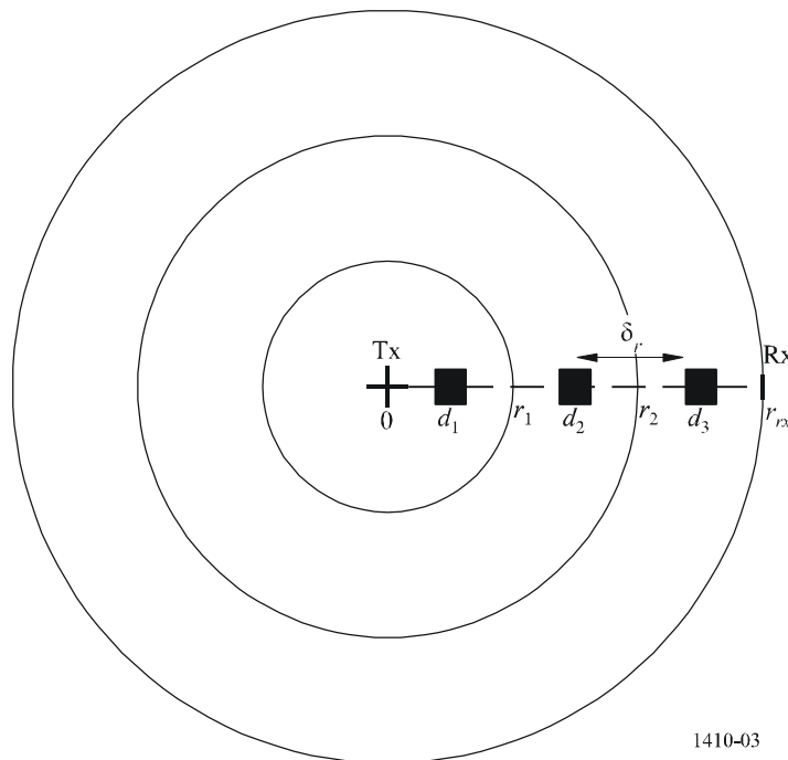
Situación de los edificios con respecto al Receptor (Rx), a una distancia, r_{rx} del Transmisor (Tx)
