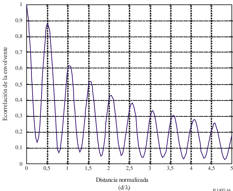
Correlación espacial resultante
