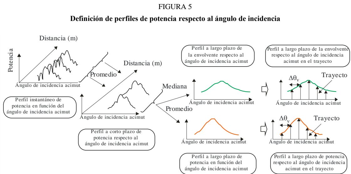
a) Definición de perfiles de potencia respecto del ángulo de incidencia acimut
