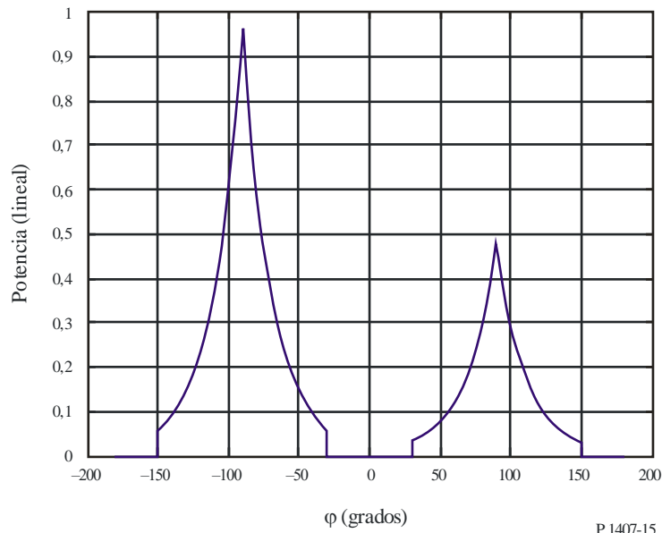
Función Laplaciana truncada ideal aplicada al espectro potencia-acimut (PAS)
