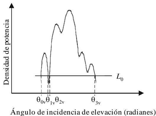
b) Potencia total del perfil de potencia del ángulo de incidencia de elevación
