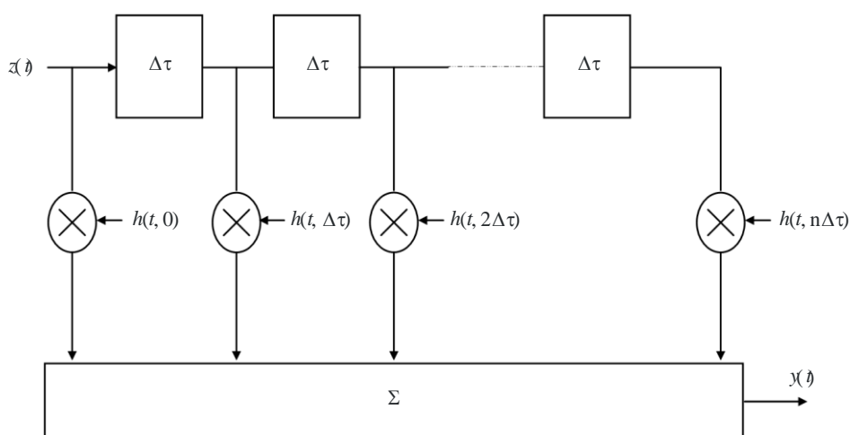
FIGURA 18B Modelo de multitrayecto con línea de retardo con derivación
