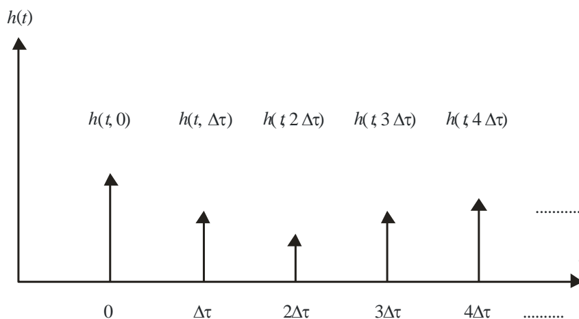
FIGURA 18A Ejemplo de multitrayecto utilizado para generar el canal
