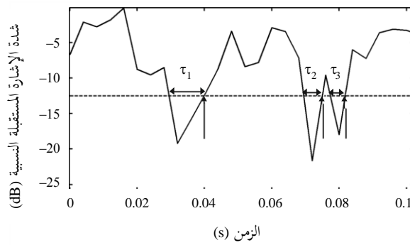
شدة الإشارة المستقبلية مقابل الزمن
