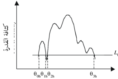
أ) القدرة الإجمالية للمقطع الجانبي لقدرة زاوية السمّت للورود
