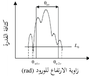
ب) النافذة الزاوية في الارتفاع
