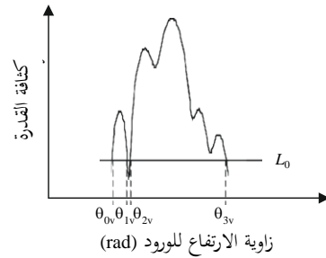
ب) القدرة الإجمالية للمقطع الجانبي لقدرة زاوية الارتفاع للورود
