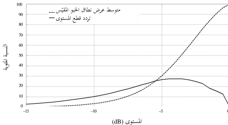
متوسط عرض نطاق الخبو المعايير وتردد قطع المستوى
