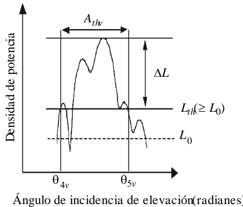
b) Intervalo angular de elevación
