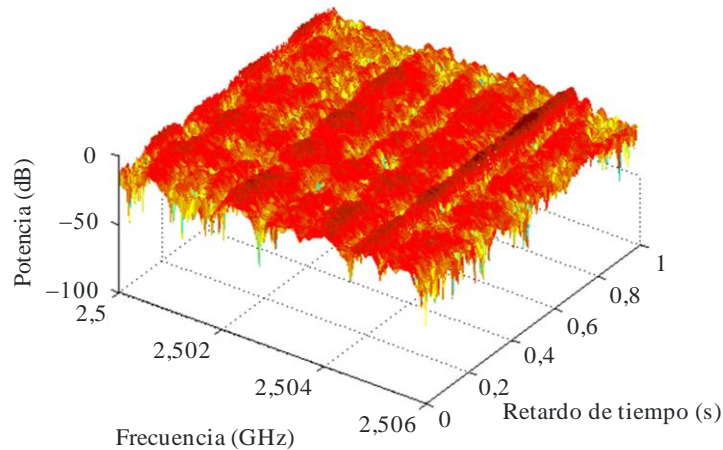
FIGURA 12 Función de respuesta en frecuencia variable en el tiempo a pequeña escala
