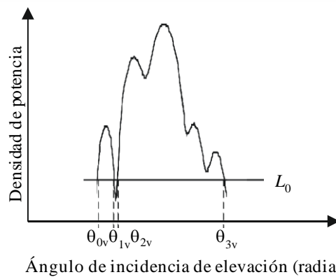
b) Potencia total del perfil de potencia del ángulo de incidencia de elevación
