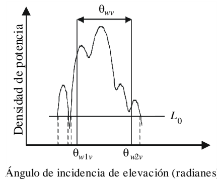
b) Ventana angular de elevación
