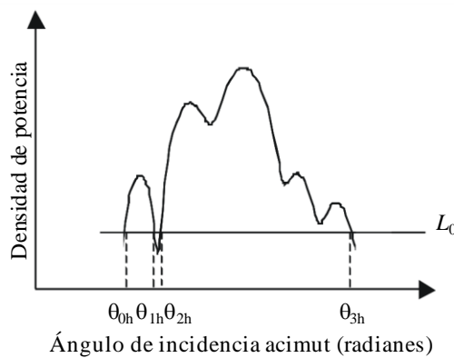
a) Potencia total del perfil de potencia del ángulo de incidencia acimut
