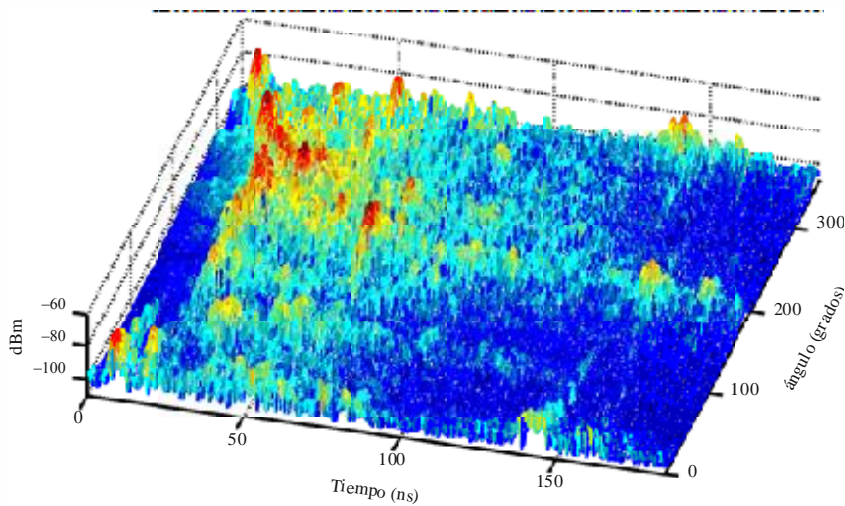
FIGURA 11 Perfiles del retardo de potencia direccional
