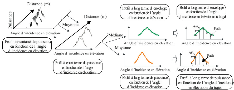
b) Définition des profils de puissance en fonction de l'angle d'incidence en élévation
