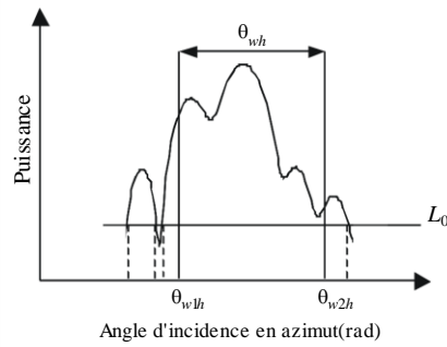
a) Fenêtre angulaire en azimut
