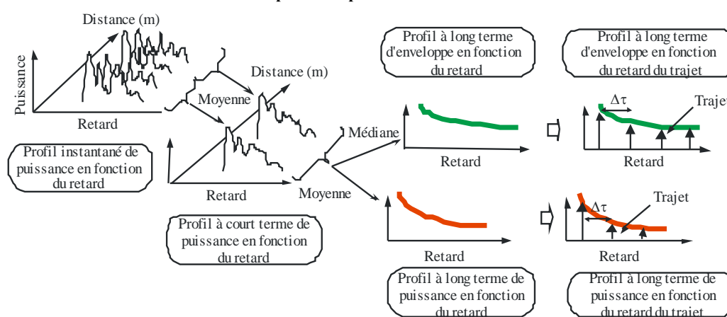
Définition des profils de puissance en fonction du retard
