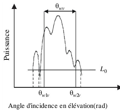
b) Fenêtre angulaire en élévation
