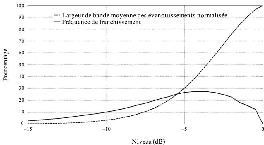
FIGURE 14 Largeur de bande moyenne des évanouissements normalisée et fréquence de franchissement
