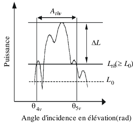
b) Intervalle angulaire en élévation
