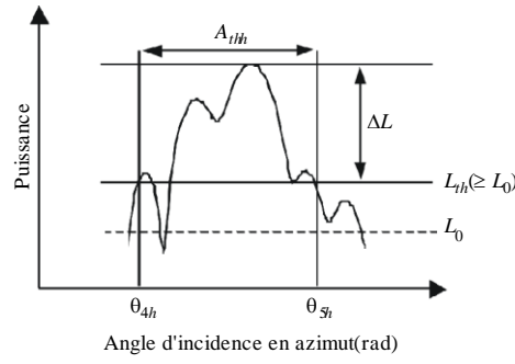
a) Intervalle angulaire en azimut
