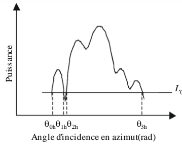
a) Puissance totale du profil de puissance en fonction de l'angle d'incidence en azimut
