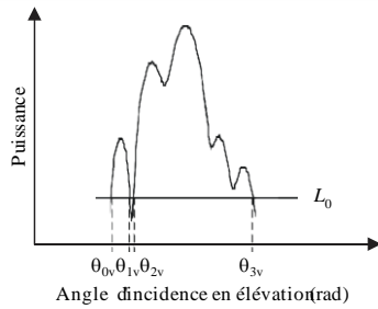
b) Puissance totale du profil de puissance en fonction de l'angle d'incidence en élévation
