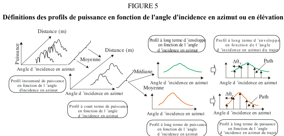
a) Définition des profils de puissance en fonction de l'angle d'incidence en azimut
