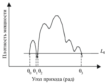
РИСУНОК 5 Общая мощность
