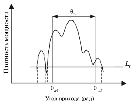
Угловое окно
