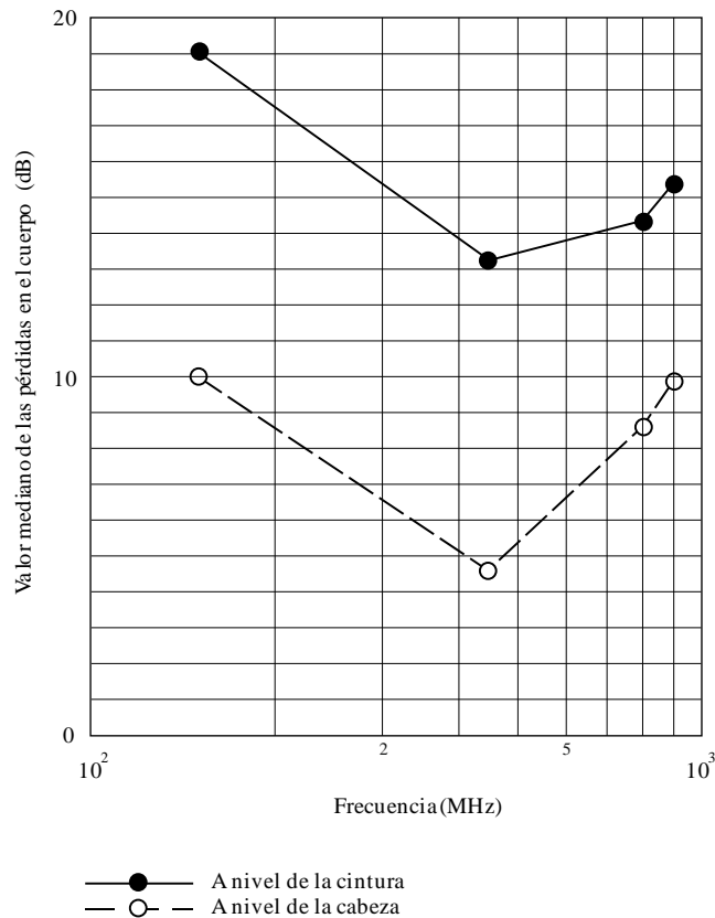
FIGURA 2 Pérdidas en el cuerpo típicas – Transceptor portátil
