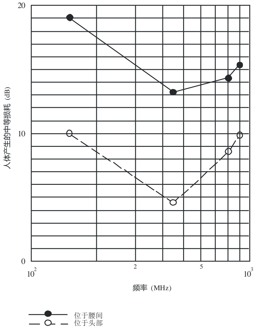
图2 人体产生的典型损耗—便携式收发器
