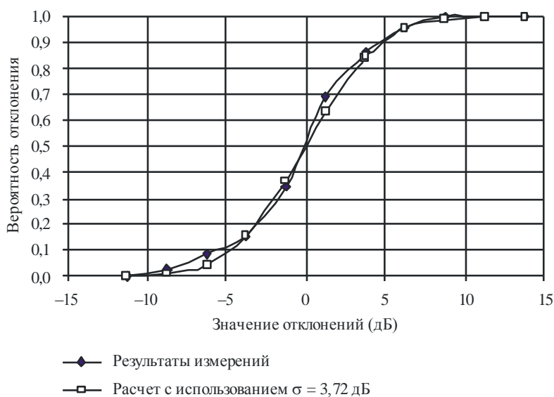
РИСУНОК 5 Закон распределения отклонений
