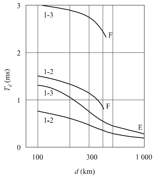
FIGURE 4 Retard réciproque des signaux transmis par l'onde ionosphérique pour différents nombres de bonds
