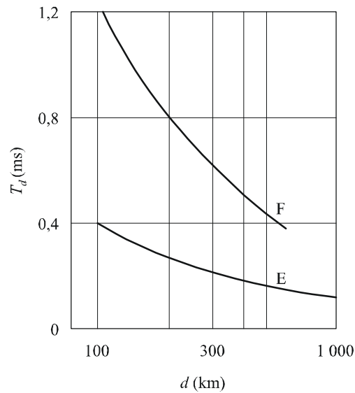
FIGURE 3 Retard relatif du signal transmis par l'onde ionosphérique par rapport au signal transmis par l'onde de sol
