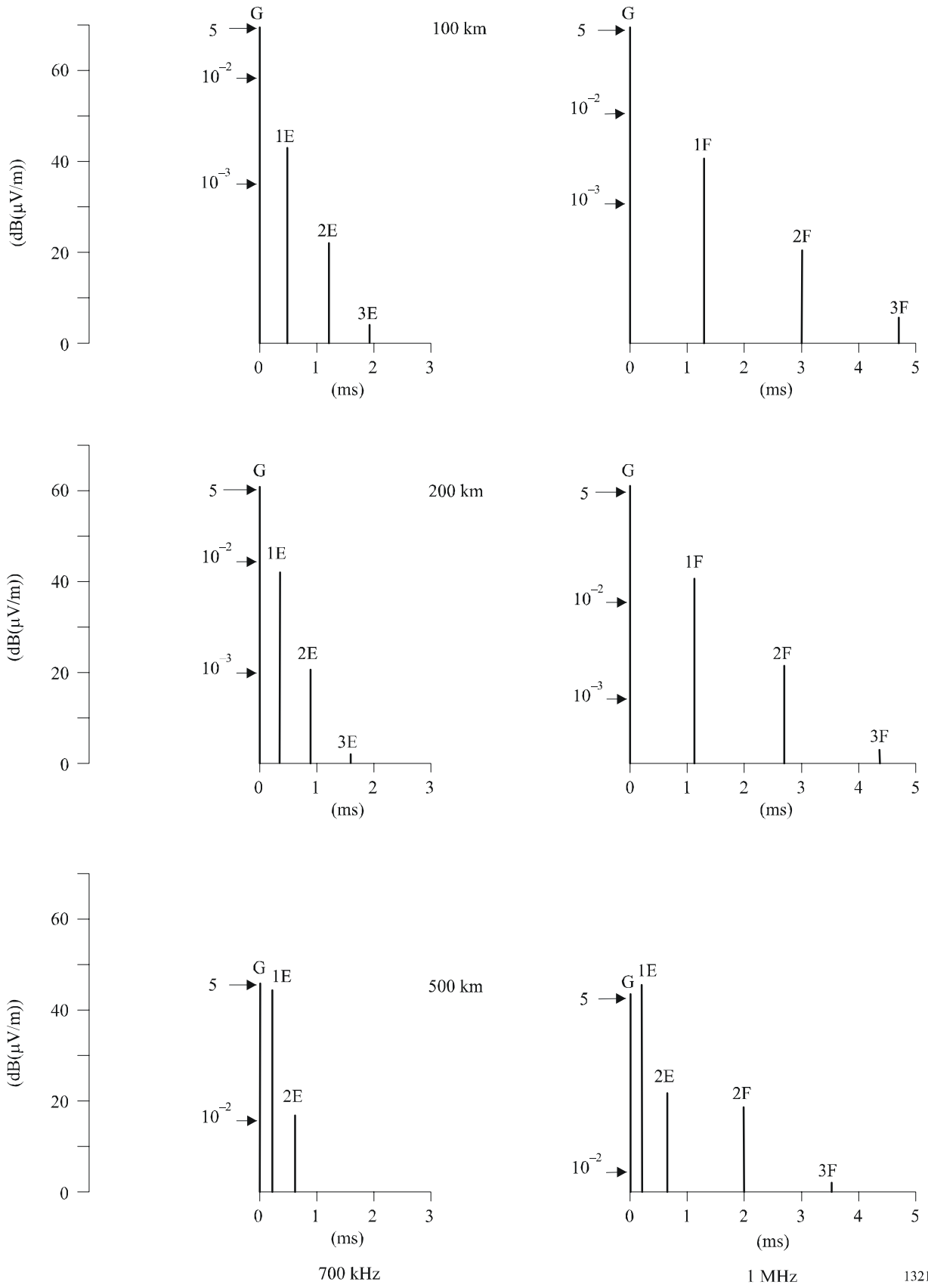
FIGURA 2 Ejemplos de dispersión del retardo en el tiempo
