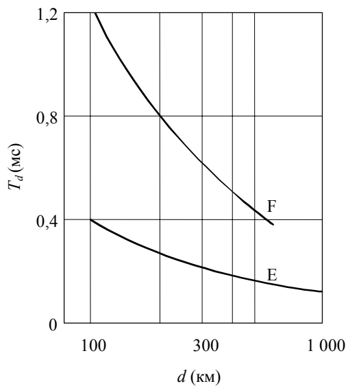
РИСУНОК 3 Задержка сигнала пространственной волны относительно сигнала земной волны
