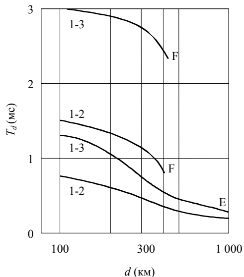
РИСУНОК 4 Общая задержка сигналов, распространяющихся посредством пространственной волны, для различного числа скачков
