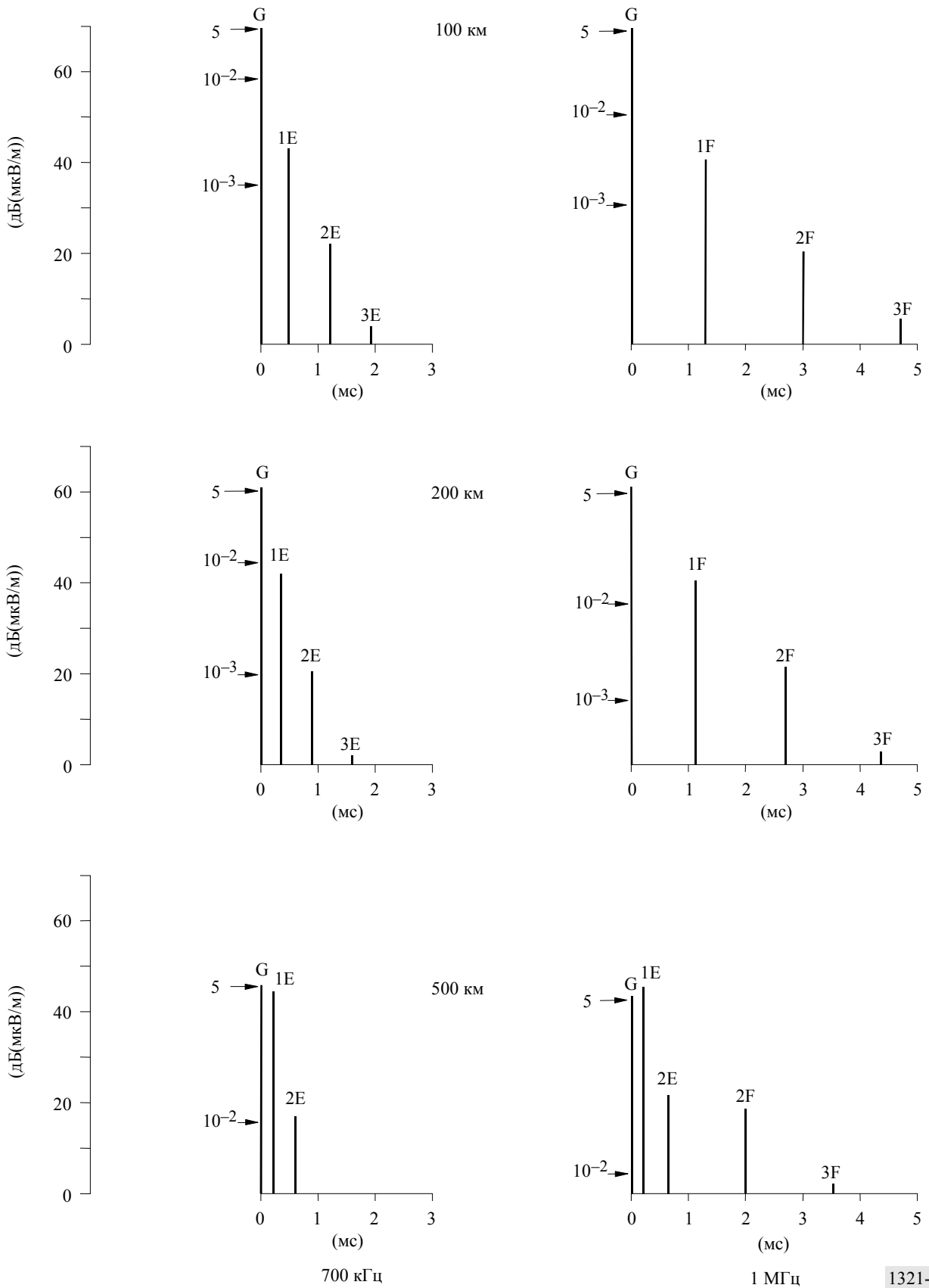
РИСУНОК 2 Примеры разброса временных задержек
