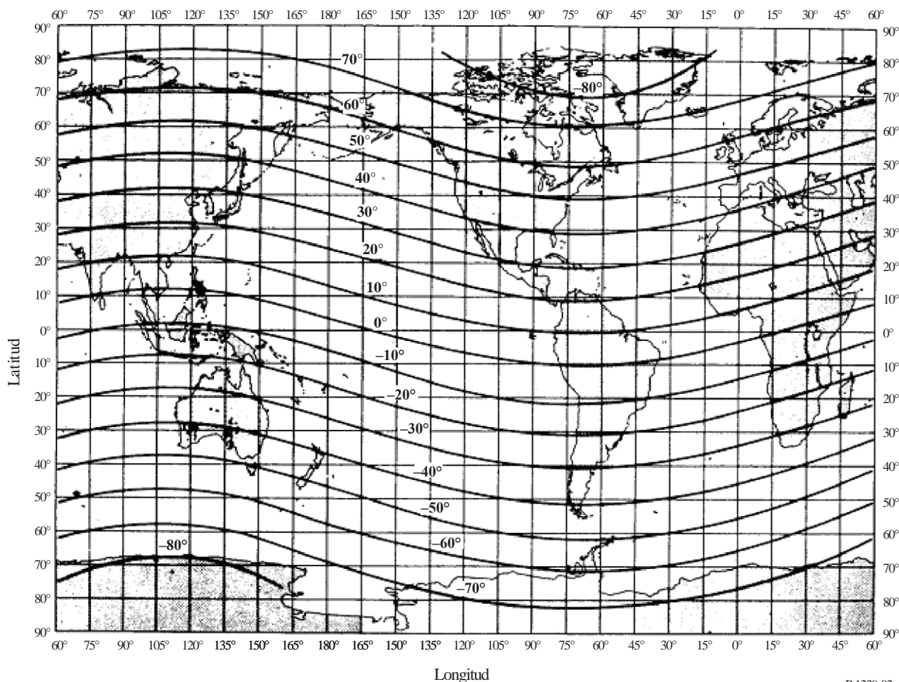
FIGURA 2 Latitudes geomagnéticas
