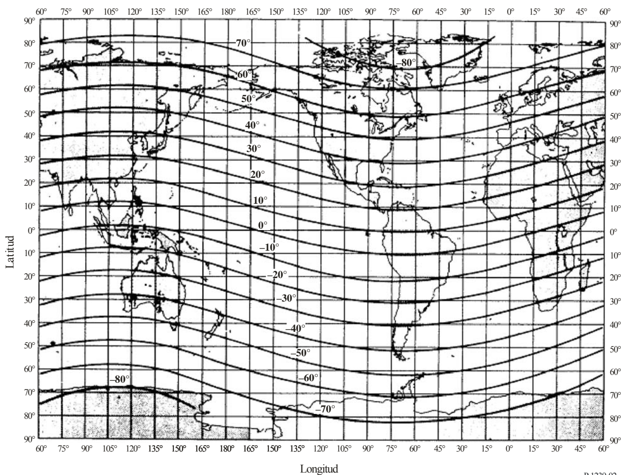
FIGURA 2 Latitudes geomagnéticas
