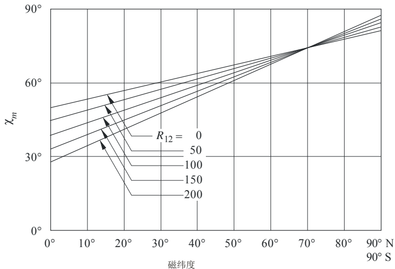
\chi_m 随地磁纬度和 R_{12} 的变化
