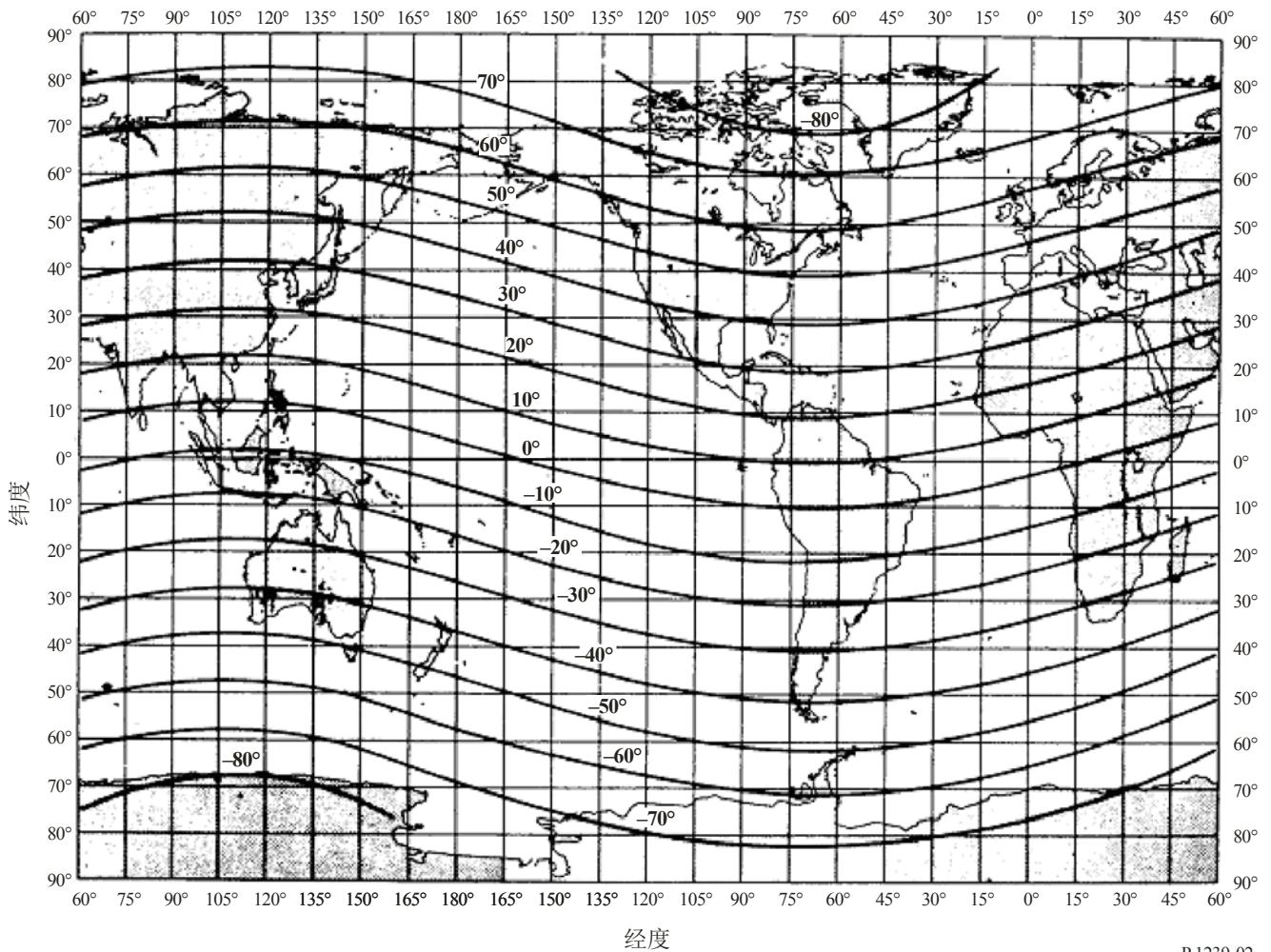
图2 地磁纬度
