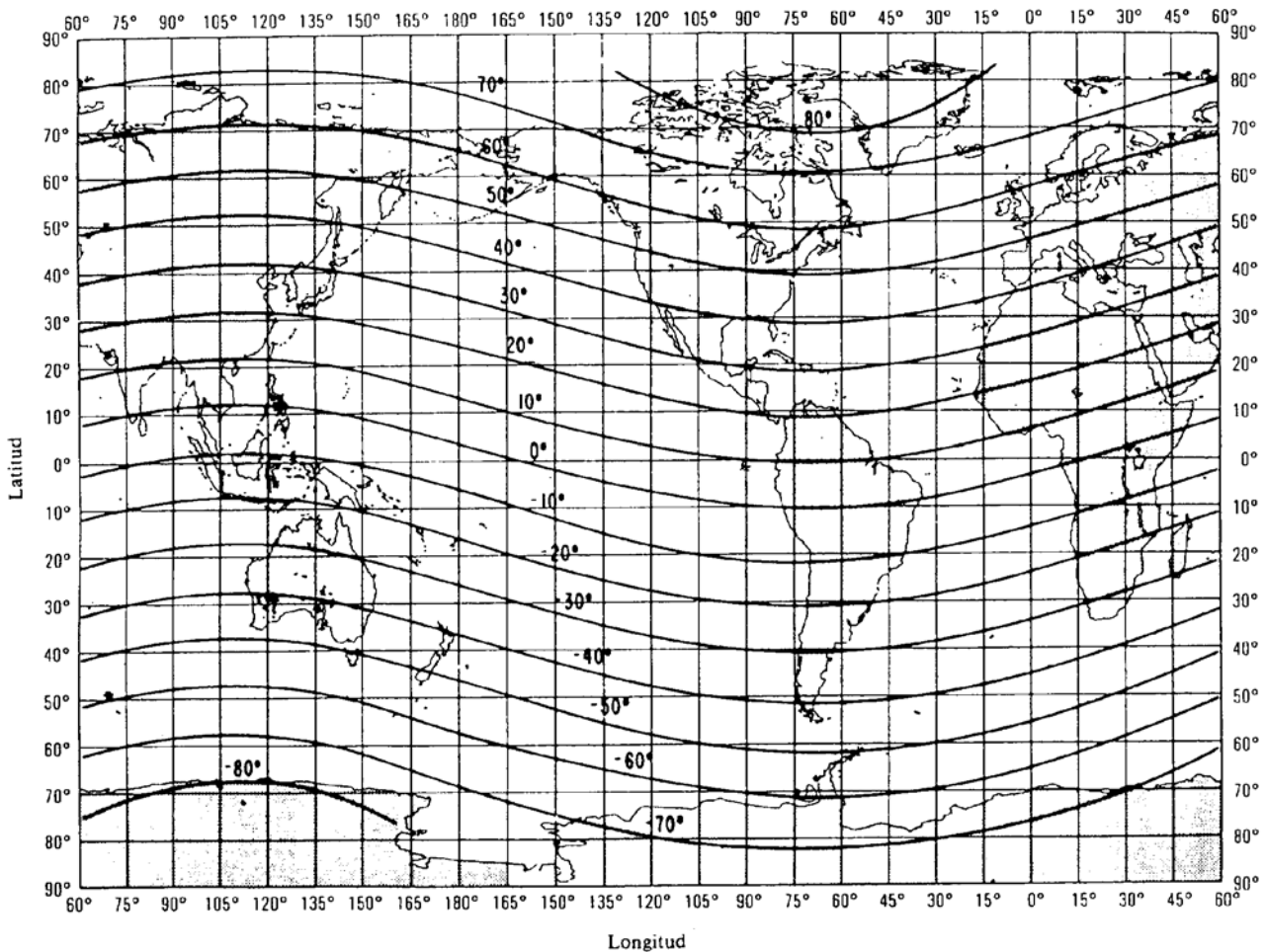
FIGURA 2 Latitudes geomagnéticas
