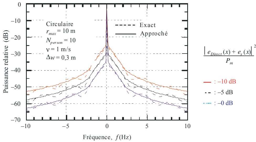
Spectre de puissance dans une pièce circulaire
