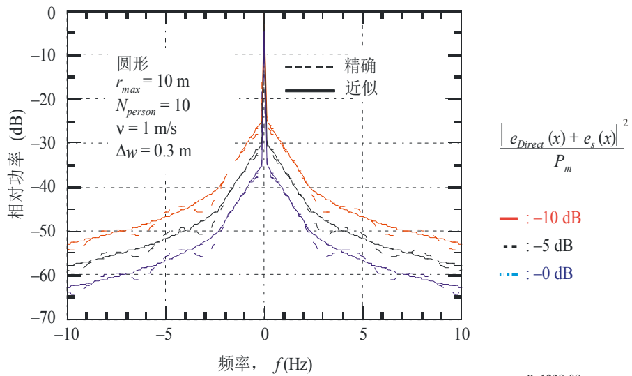
图 8 圆形方向中的功率谱
