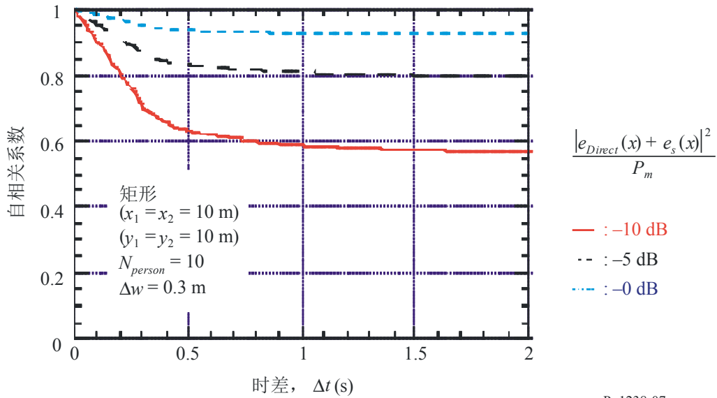
圆形房间中接收电平的自相关系数
