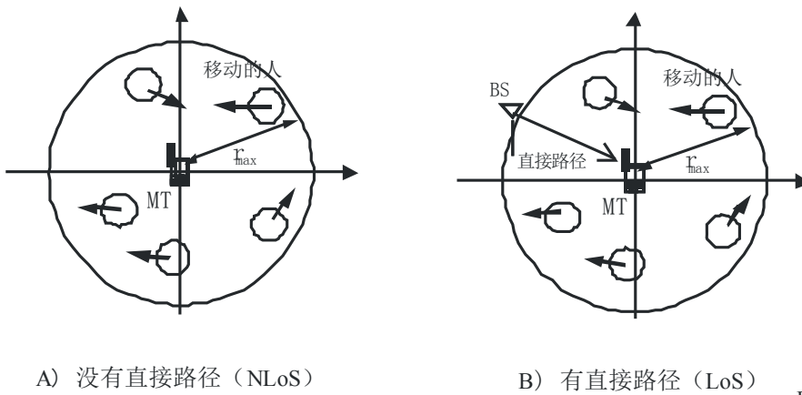
图5 圆形房间布局
