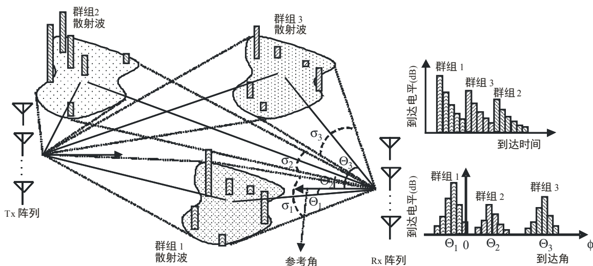
图2 群组模型图
