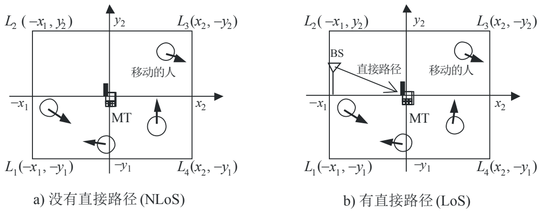
图4 矩形房间的布局
