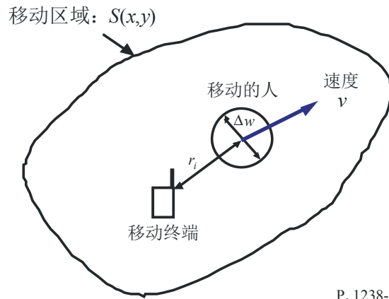
图3 系统模型
