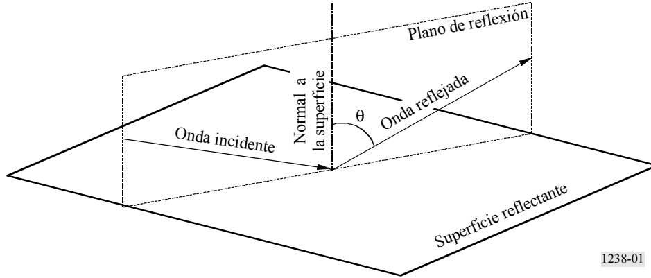
FIGURA 1 Geometría para calcular las características de la reflexión
