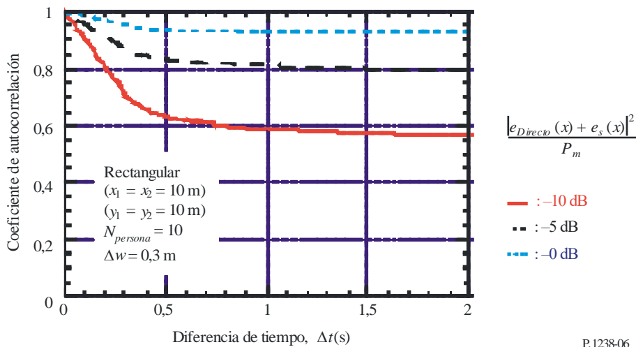
Coefficiente de autocorrelaci3n del nivel recibido en una sala circular
