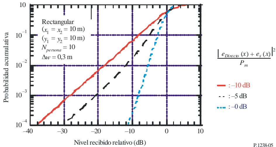
Probabilidad acumulativa del nivel recibido en una sala circular
