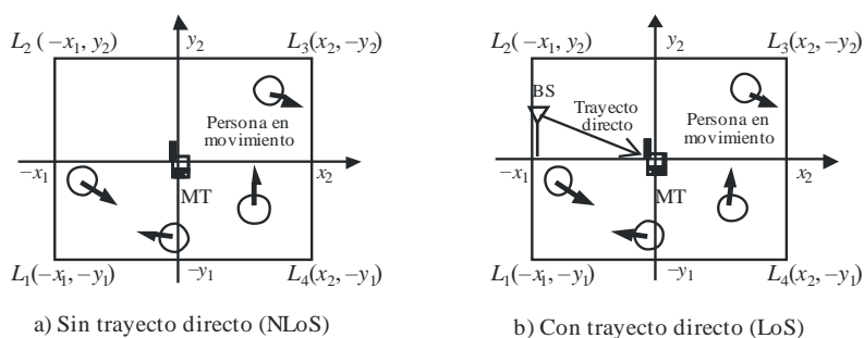
FIGURA 3 Disposición en una habitación rectangular
