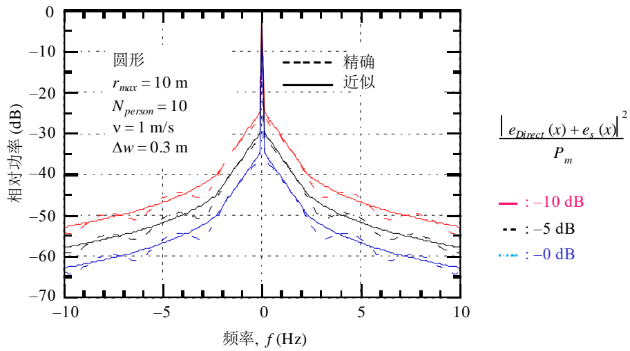
圆形房间中的功率谱
