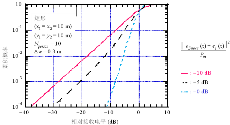
圆形房间接收电平的累积概率
