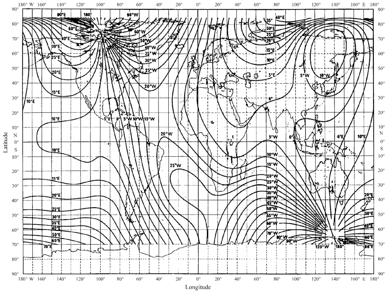
FIGURE 6 Carte de déclinaison magnétique (pour 1975,0)
