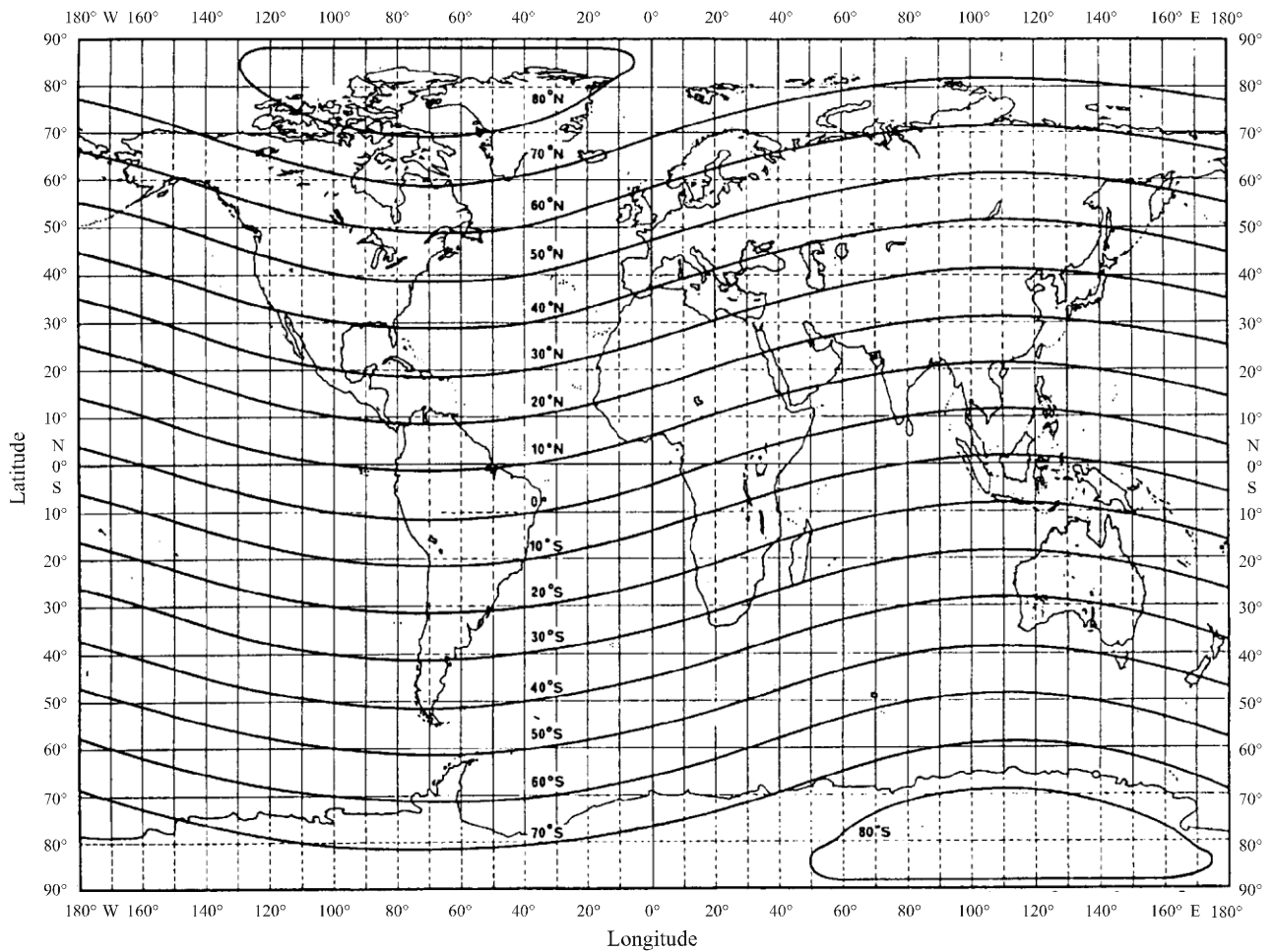
FIGURE 10 Latitudes géomagnétiques
