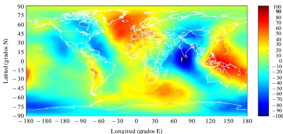
FIGURA 5 EGM2008 (m)
