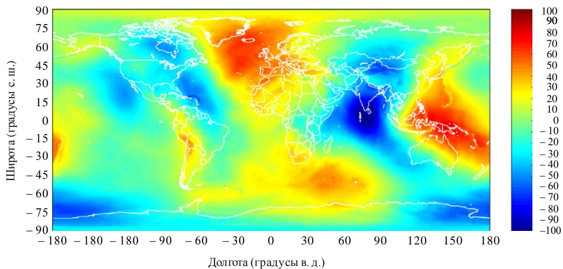
РИСУНОК 5 EGM2008 (м)
