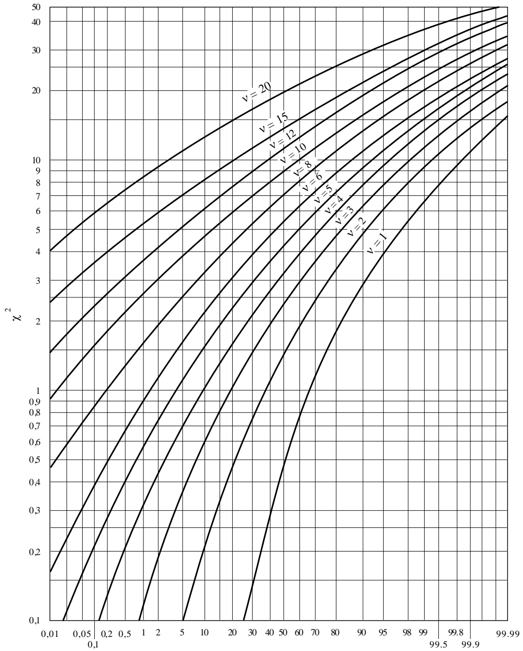
FIGURE 7 Distribution de probabilité en \chi^2
