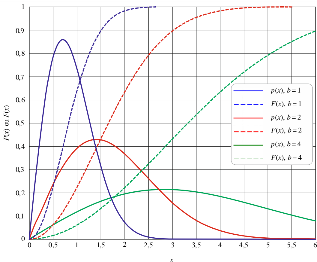
FIGURE 2 Distribution de probabilité de Rayleigh
