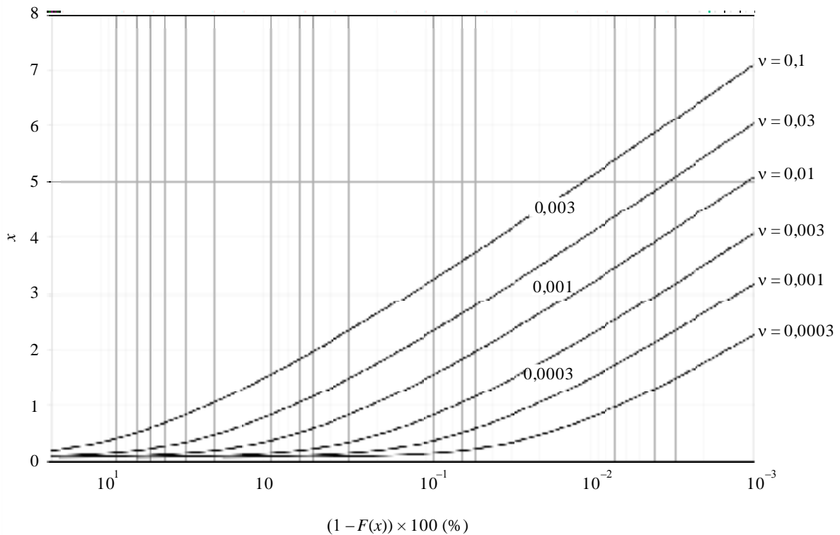
FIGURE 5 Distribution de probabilité gamma \alpha = 1, v \leq 0,1
