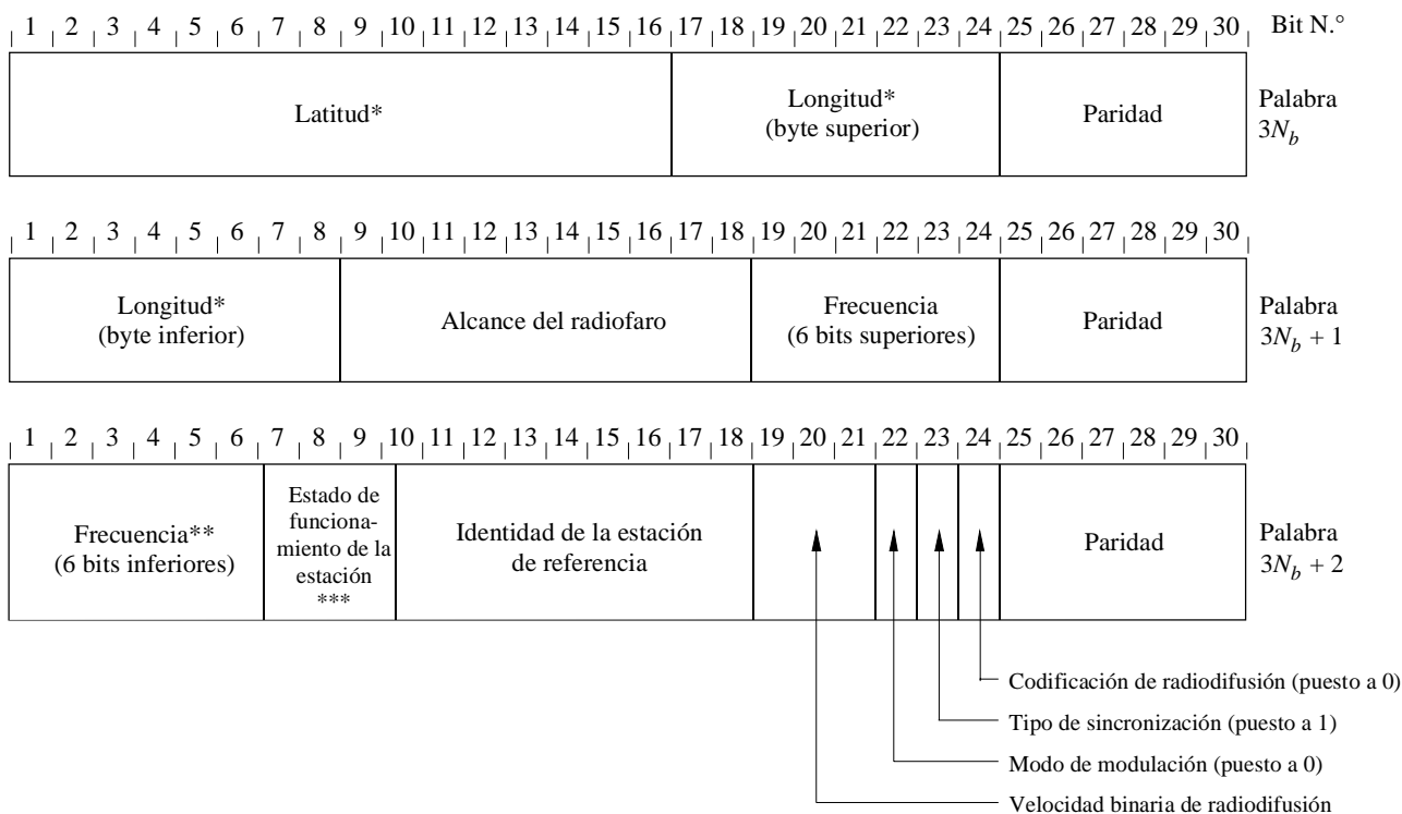
FIGURA 11 Formato de mensajes de tipo 35 Informaciones sobre las transmisiones del radiofaro (GLONASS)
