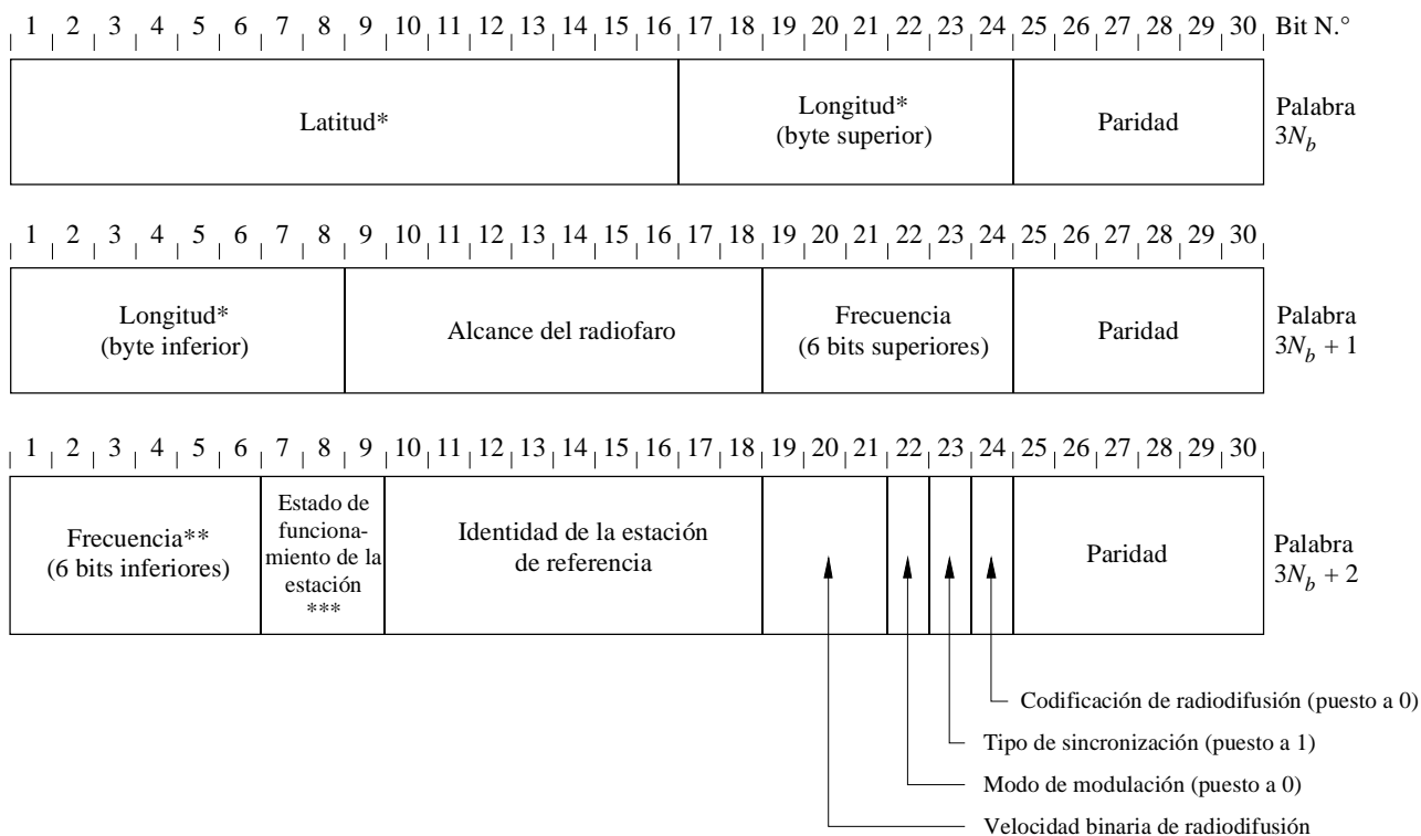
FIGURA 6 Formato de mensajes de tipo 7 Informaciones sobre las transmisiones del radiofaro (GPS)
