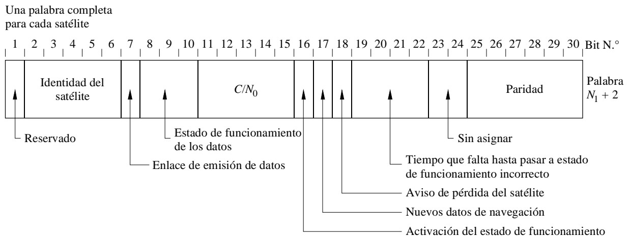
FIGURA 5 Formato de los mensajes de tipo 5 Estado de funcionamiento de la constelación (GPS) (véase el Cuadro 3)
