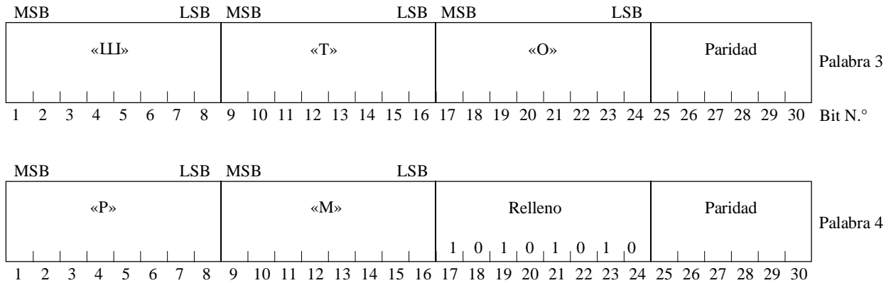
FIGURA 12 Tipo de mensajes 36 Mensajes especiales GLONASS
